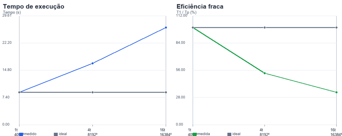
Imagem 4: Teste de escalabilidade fraca
