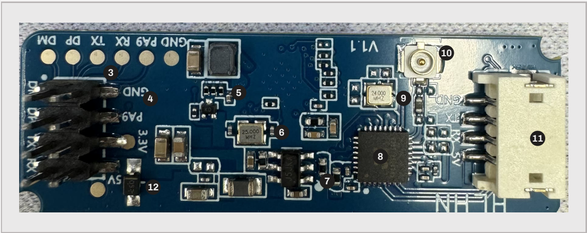
Obr. 8 HLK-LD2450 ze strany součástek. Čísla odkazují na tabulku pod obrázkem; radarový čip leží na druhé straně desky za krystalem 6.
