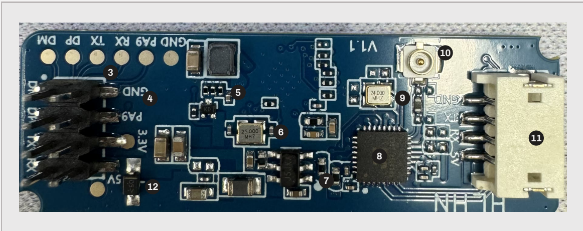
Obr. 8 HLK-LD2450 ze strany součástek. Čísla odkazují na tabulku pod obrázkem; radarový čip leží na druhé straně desky za krystalem ⑥.
