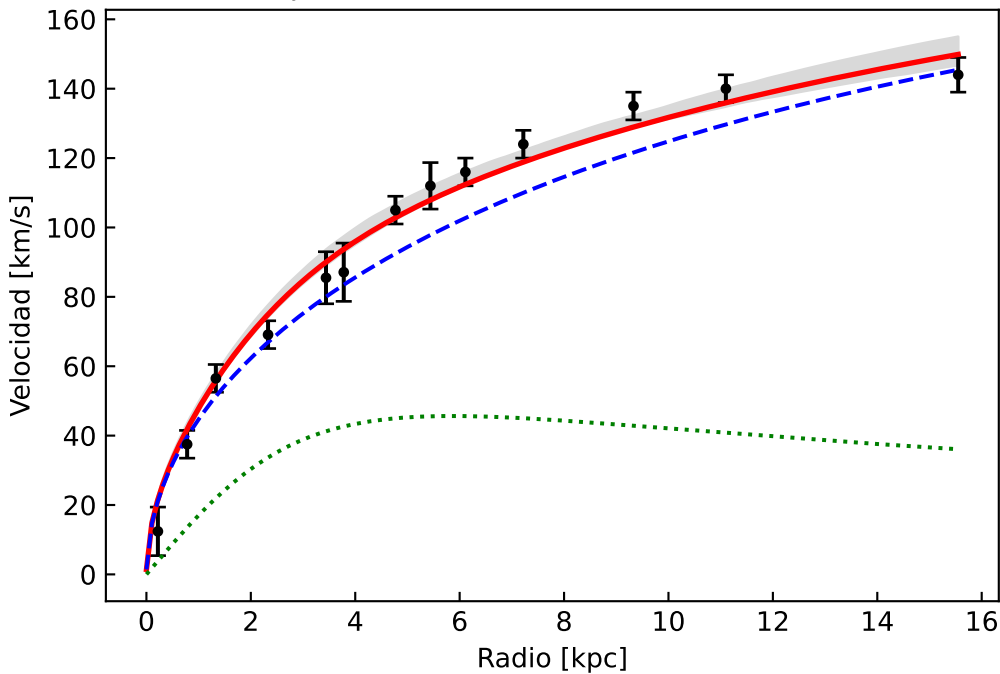
Ajuste curva de rotación de F571-8
