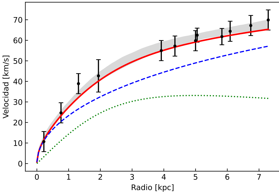
Ajuste curva de rotación de F583-4
