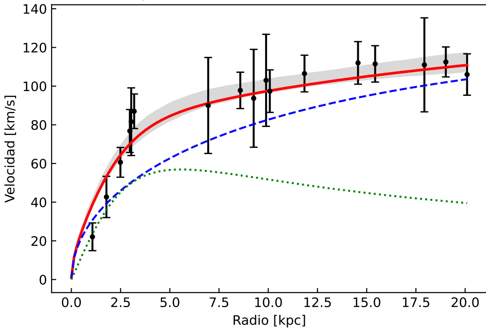
Ajuste curva de rotación de F563-1
