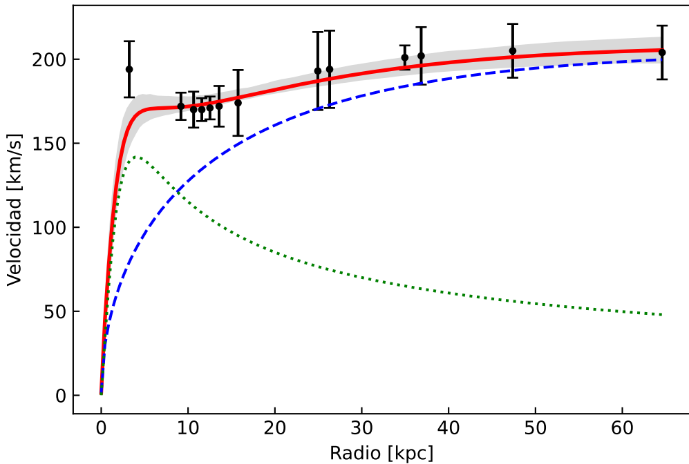
Ajuste curva de rotación de UGC06614
