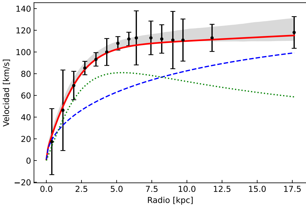
Ajuste curva de rotación de F568-V1
