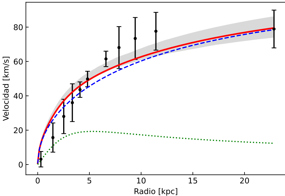
Ajuste curva de rotación de UGC05750
