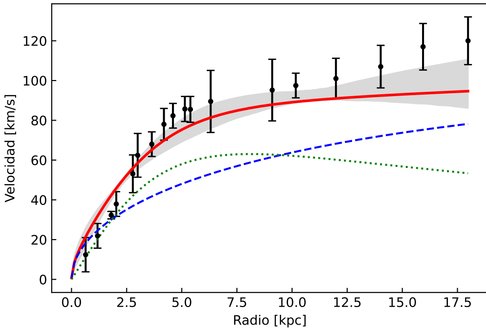
Ajuste curva de rotación de F568-3
