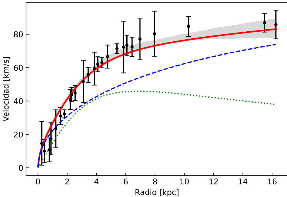
Ajuste curva de rotación de F583-1
