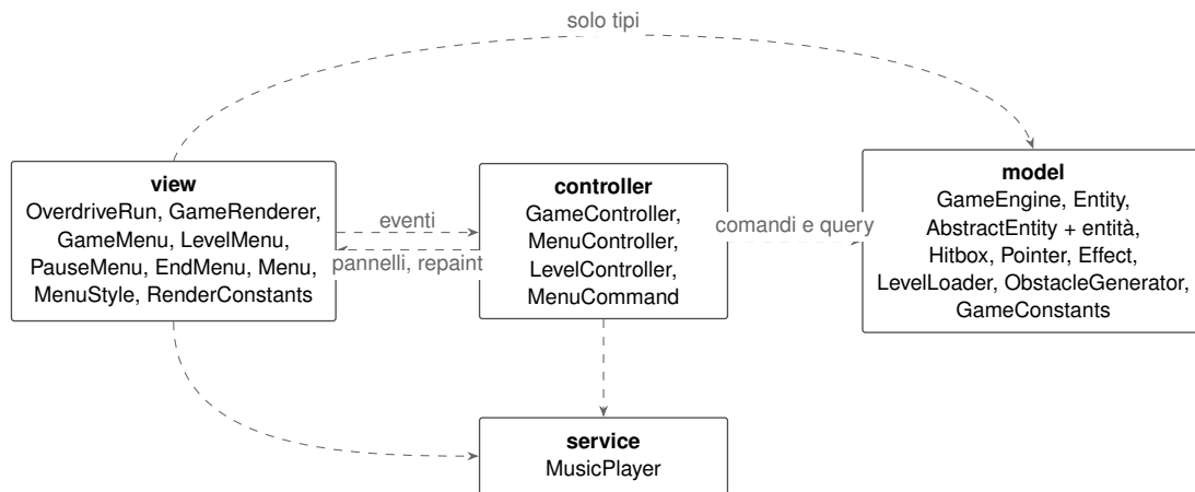
Figura 2.1: Dipendenze fra i package. Il modello è l'unico senza dipendenze uscenti.
