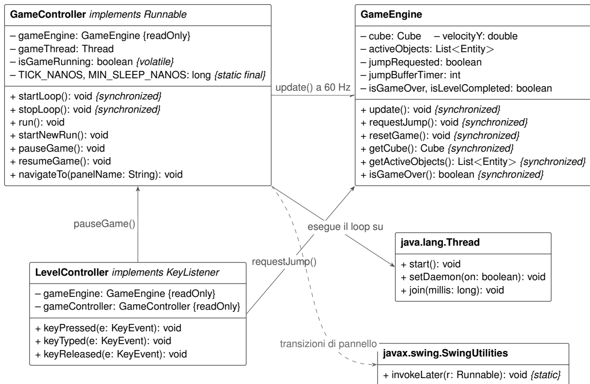
Figura 2.4: Ciclo di gioco e interazione fra thread.
