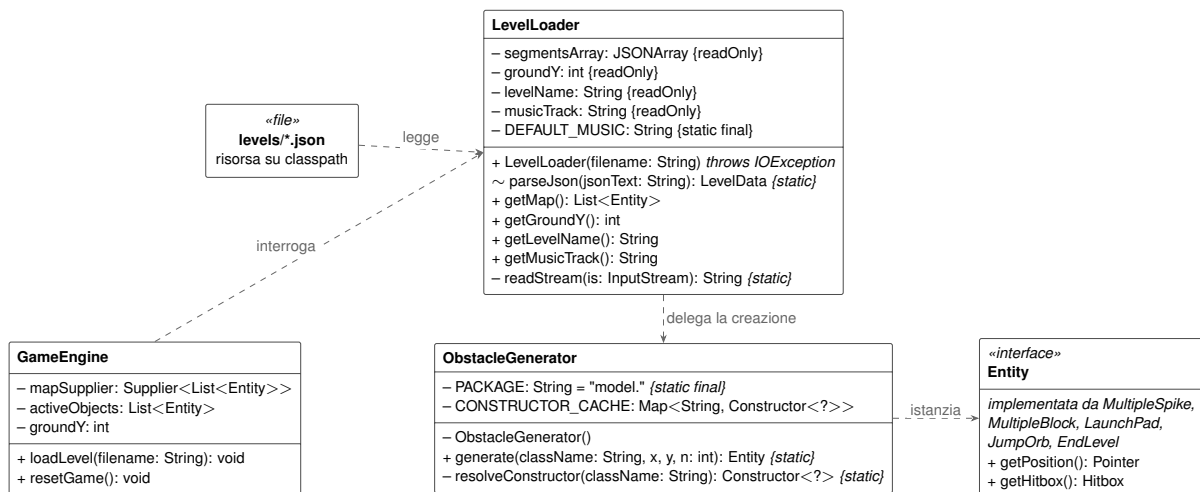
Figura 2.3: Caricamento di un livello e creazione riflessiva delle entità.
