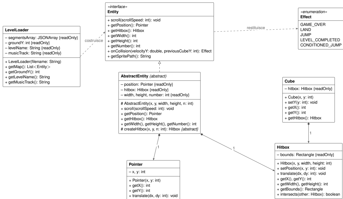
Figura 1.2: Modello del dominio: entità del problema, con la struttura che assumono nel modello dell'applicazione.
