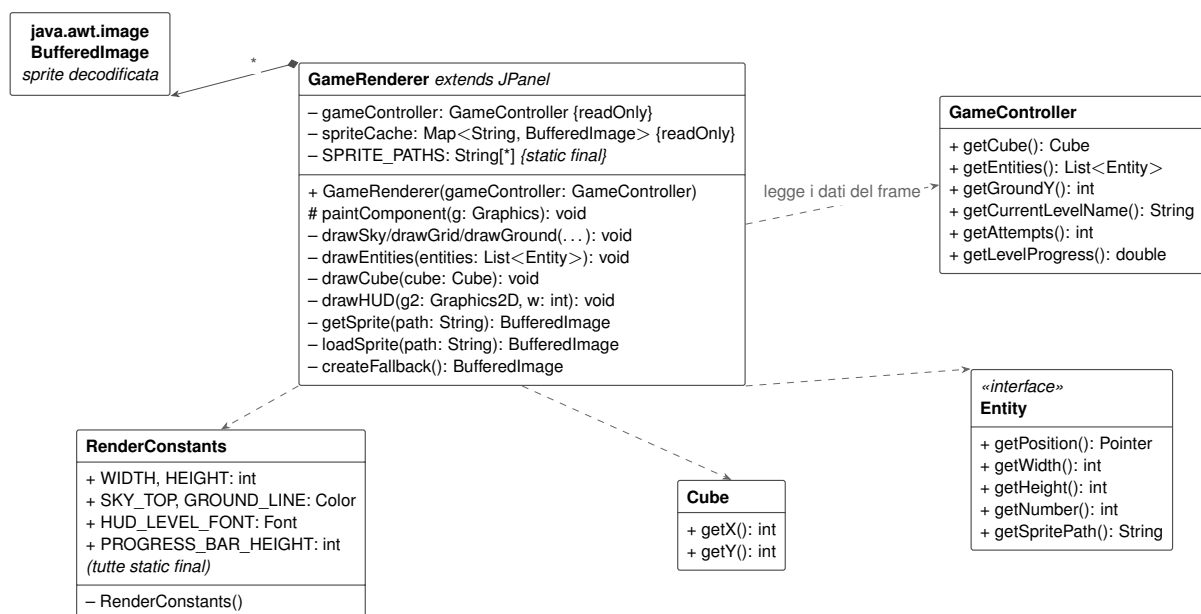
Figura 2.7: Rendering: il renderer dipende dal solo Controller.
