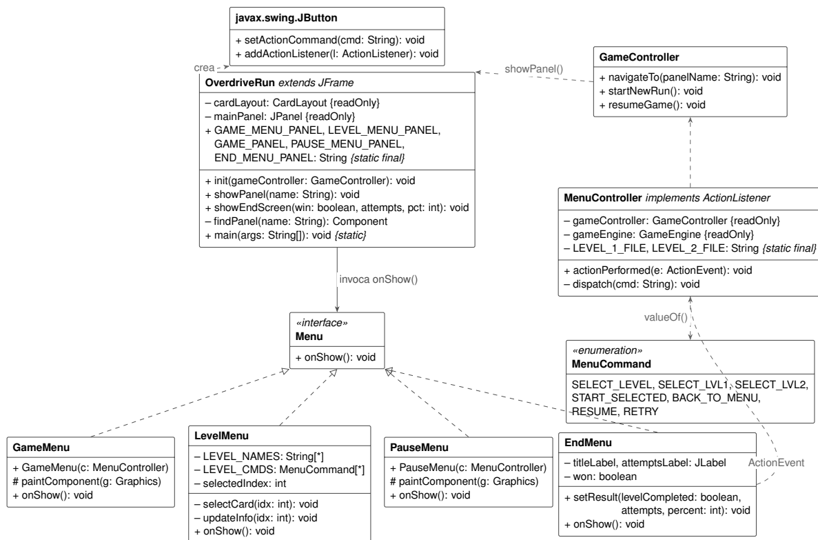
Figura 2.5: Navigazione fra le schermate e dispatch dei comandi di menu.
