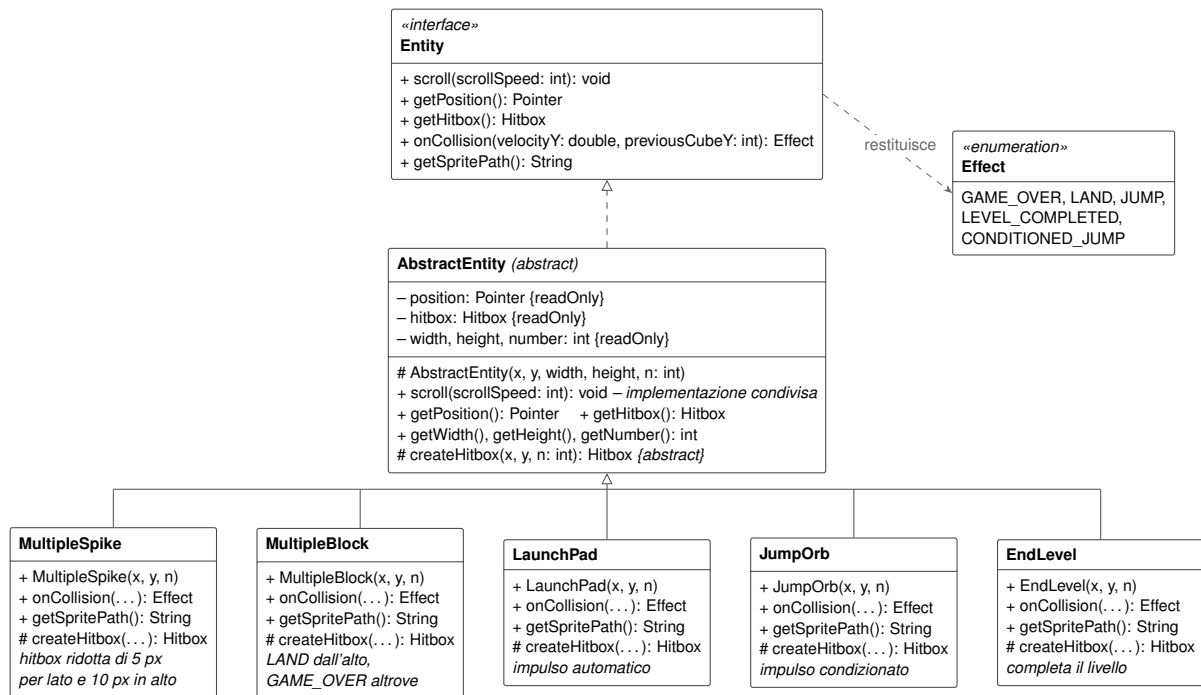
Figura 2.2: Gerarchia delle entità di gioco.
