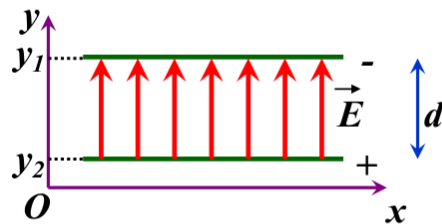
Figura 13.2: Campo elettrico del condensatore piano
