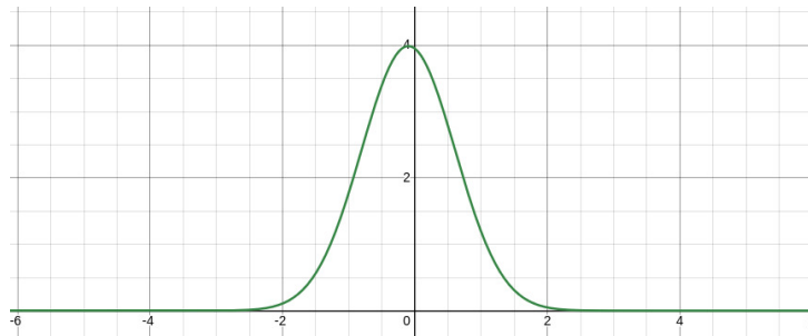
Figura 6.3: Grafico della distribuzione gaussiana
