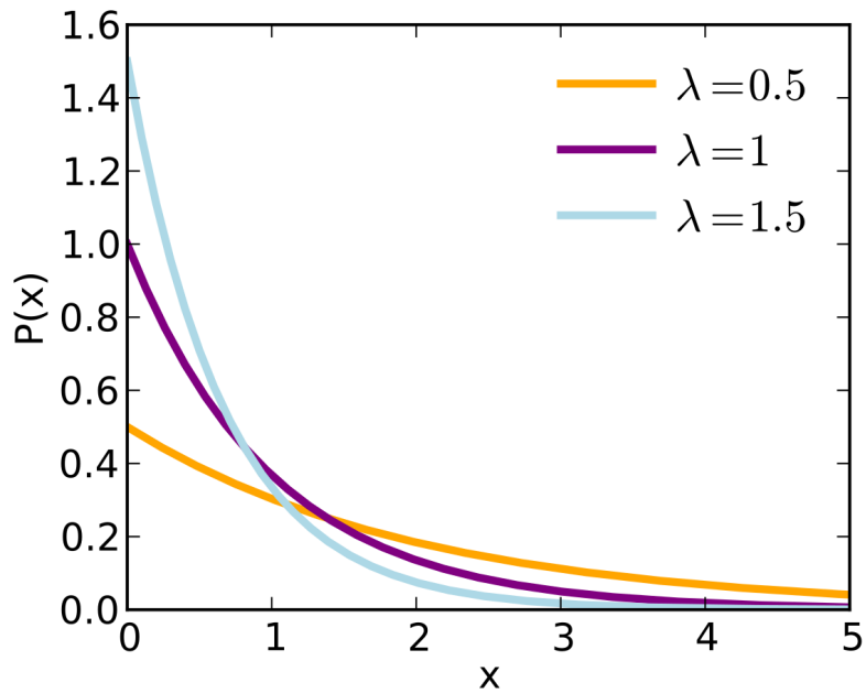
Figura 6.1: Grafico della legge della distribuzione esponenziale
