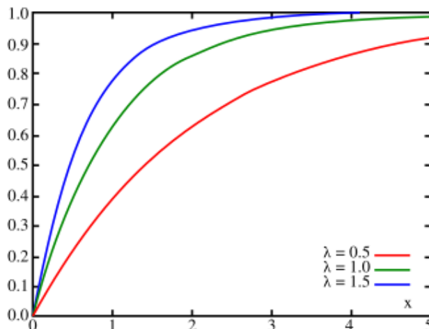
Figura 6.2: Grafico della funzione di ripartizione della distribuzione esponenziale
