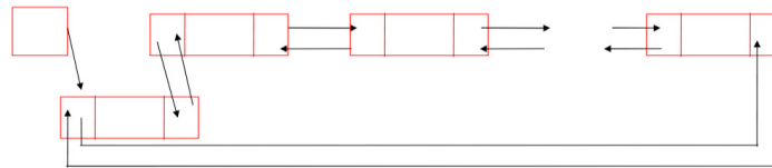
Figura 4.4: Realizzazione di una lista a doppi puntatori circolare
