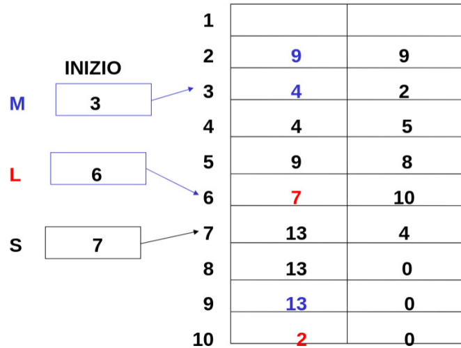
Figura 4.1: Rappresentazione di una lista mediante cursori
