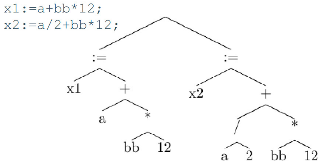
Figura 8.2: Esempio dell'albero sintattico astratto
