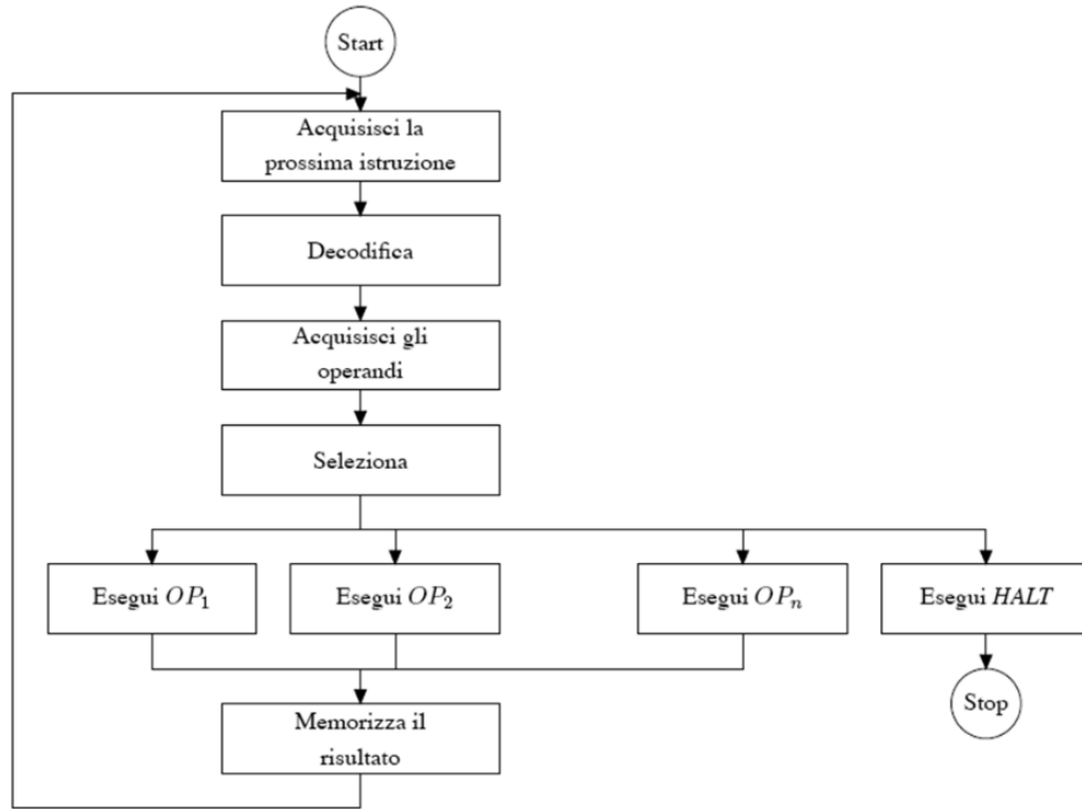
Figura 1.2: Ciclo di esecuzione di un generico interprete
