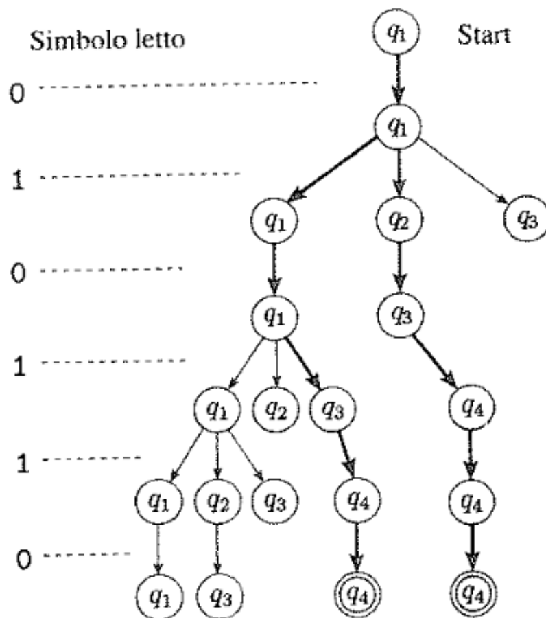
Figura 1.1: La computazione dell'automa precedente su 010110
