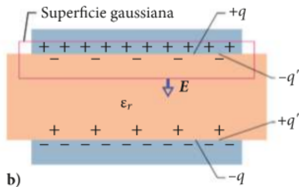
Figura 14.1: Un condensatore piano con una lastra di dielettrico inserita
