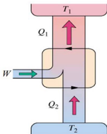
Figura 9.7: Macchina refrigerante
