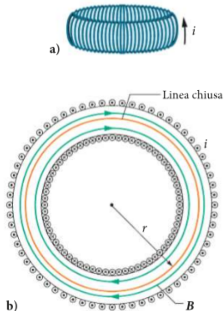
Figura 16.2: a) Un toroide percorso da corrente i . b) Una sezione trasversale del toroide
