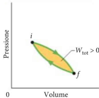
Figura 9.5: Un ciclo termodinamico
