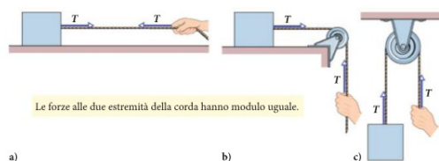
Figura 6.2: La corda è in tensione. Se la sua massa è trascurabile, la corda tira il corpo e la mano con una forza \vec{T} , anche se la corda scorre attorno a una carrucola priva di massa e di attrito
