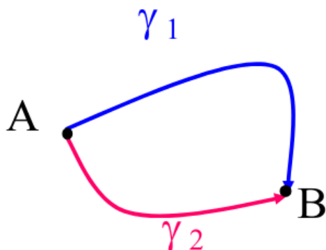
Figura 7.1: Traiettoria chiusa
