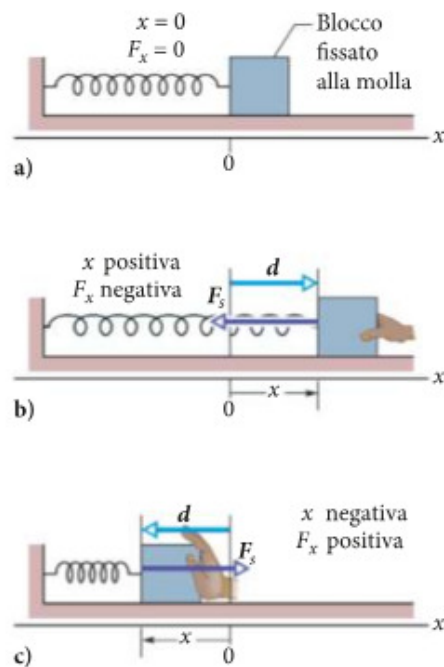
Figura 6.1: La prima figura mostra la molla in stato di riposo. La seconda figura mostra l'allungamento della molla verso destra. Nella terza figura la molla viene compressa verso sinistra.
