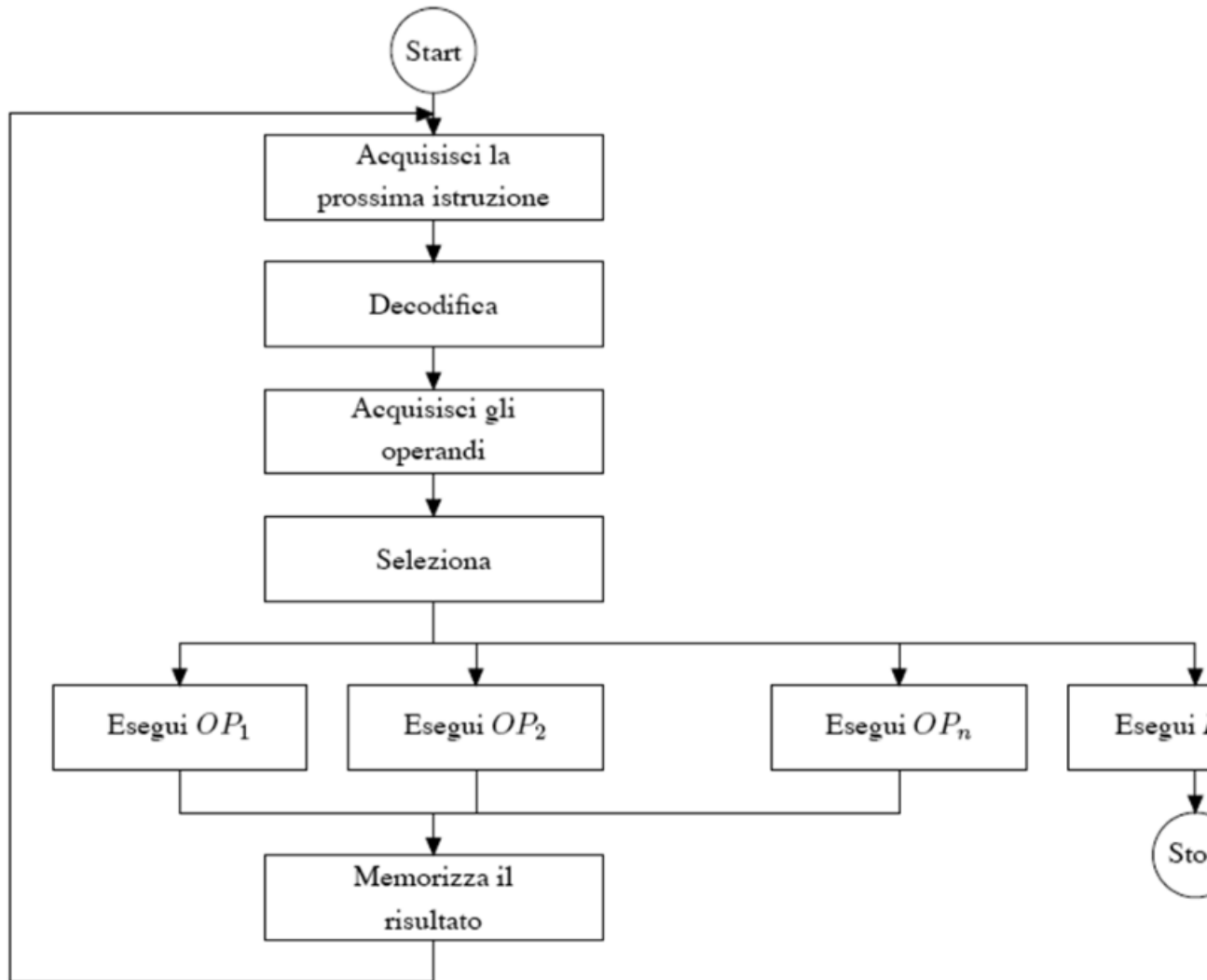
Figura 1.2: Ciclo di esecuzione di un generico interprete
