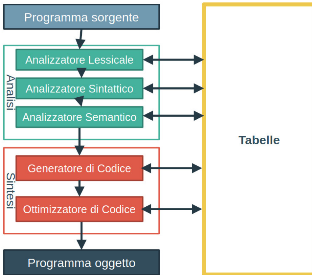
Figura 8.1: Modello funzionale di un compilatore
