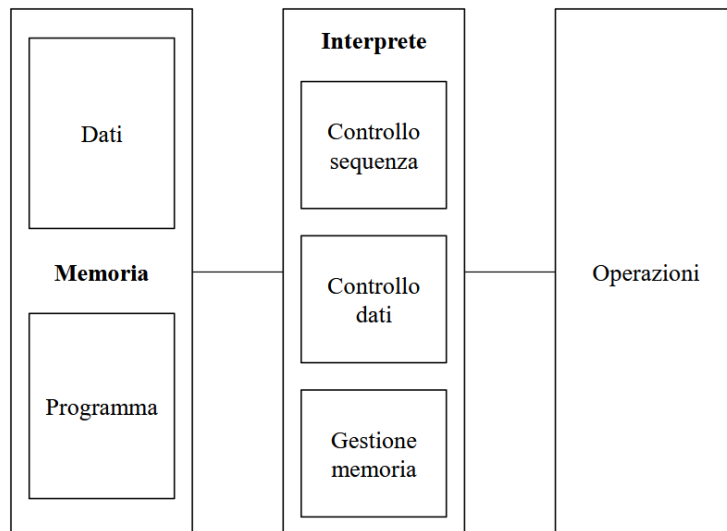
Figura 1.1: La struttura di una macchina astratta
