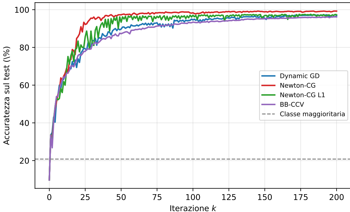
NSynth (rete neurale): accuratezza di test vs iterazioni
