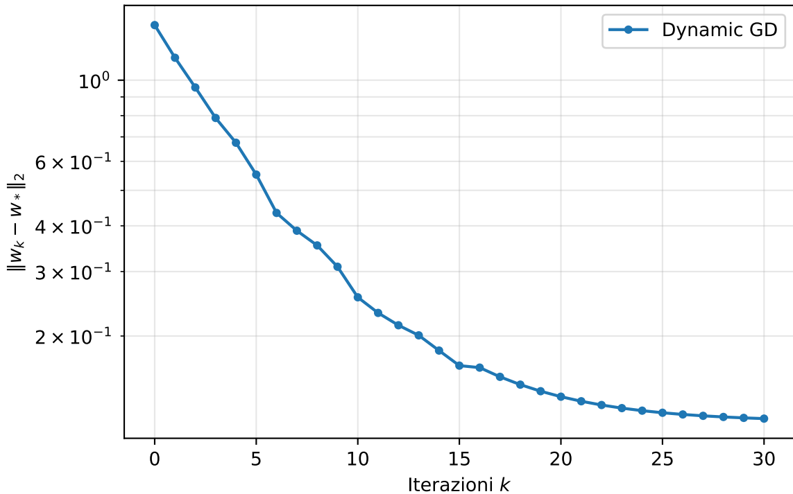
Convergenza del gradiente a campione dinamico (Wolfe + CCV)
