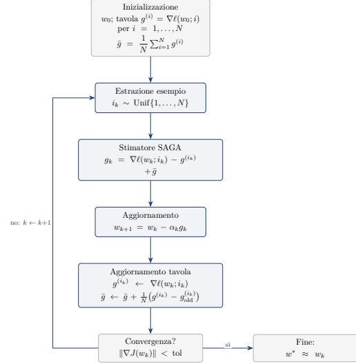
Figura D.2. Schema del metodo SAGA di Defazio, Bach e Lacoste-Julien [10]: la tavola dei gradienti g^{(i)} memorizza l'ultimo gradiente calcolato per ogni esempio ed è aggiornata a ogni iterazione; lo stimatore usa la media \bar{g} della tavola come correzione. Anche in questo caso \mathbb{E}_{i_k}[g_k] = \nabla J(w_k) e la varianza è ridotta rispetto al gradiente stocastico puro.
