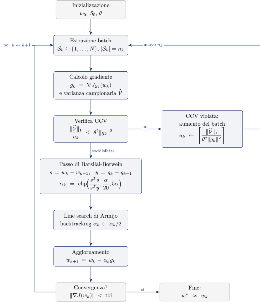
Figura E.1. Schema dell'algoritmo BB-CCV (gradiente a campione dinamico con passo di Barzilai–Borwein). Il flusso è quello del Dynamic GD (Figura 5.1): estrazione del batch S_k , calcolo di gradiente e varianza campionaria \hat{V} , verifica della CCV con eventuale aumento di n_k . La differenza è nel passo: per k > 0 si stima la curvatura di J usando solo i gradienti già calcolati, s = w_k - w_{k-1} e y = g_k - g_{k-1} , con la formula \alpha_k^{BB} = \frac{s^T s}{s^T y} di Barzilai–Borwein (per k = 0 , \alpha_0 = \alpha ); il passo è salvaguardato in [\alpha/20, 5\alpha] per la stabilità sui problemi non quadratici e rifinito da una line search di Armijo con backtracking. BB usa solo quantità già disponibili, quindi non richiede la Hessiana: negli esperimenti il metodo impiega 18 iterazioni medie (contro le 30 del GD) e sui problemi mal condizionati raggiunge precisioni 10^{-8} – 10^{-14} invece di 10^{-1} – 10^{-2} .
