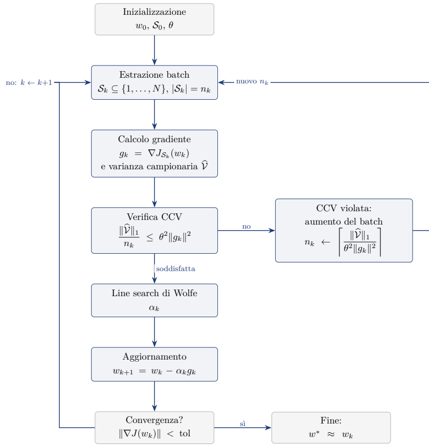
Figura 5.1. Schema dell'algoritmo con controllo della varianza campionaria (CCV): il flusso principale segue inizializzazione → estrazione batch → calcolo di gradiente e varianza → verifica della CCV → line search → aggiornamento; quando la CCV è violata la dimensione del batch viene aumentata e si ripete l'estrazione.
