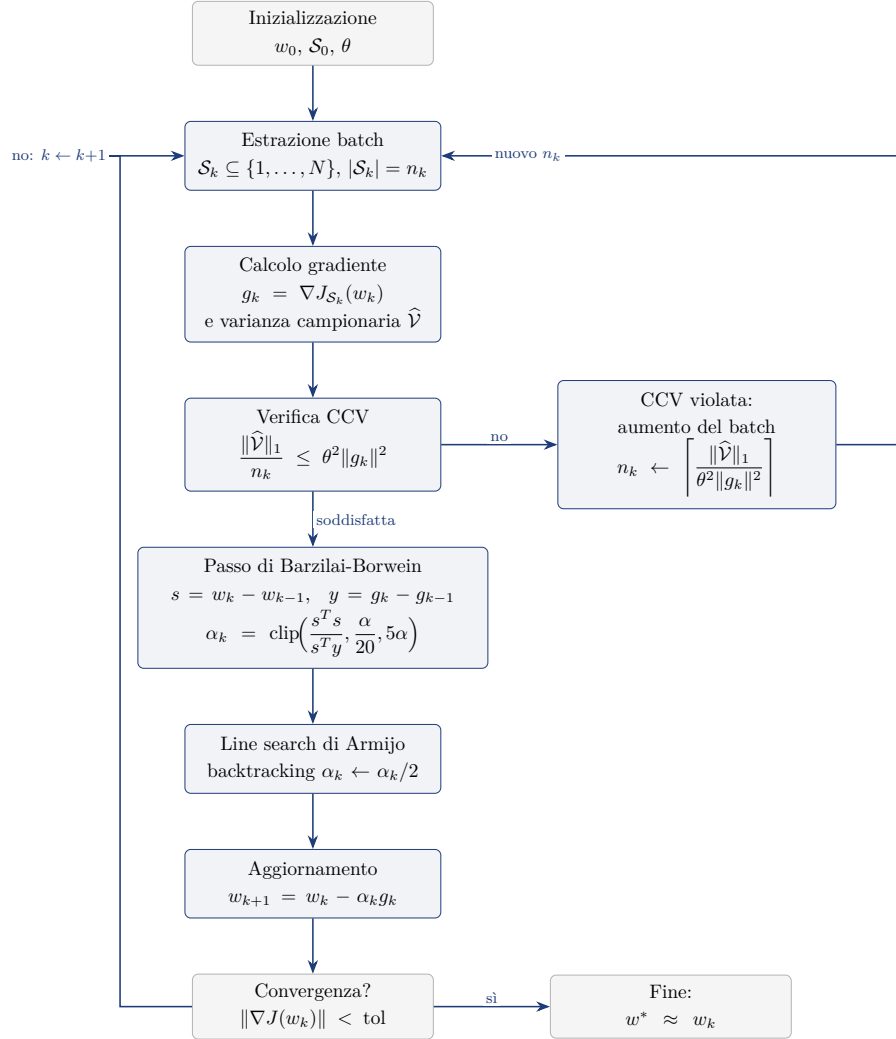
Figura E.1. Schema dell'algoritmo BB-CCV (gradiente a campione dinamico con passo di Barzilai–Borwein). Il flusso è quello del Dynamic GD (Figura 5.3): estrazione del batch S_k , calcolo di gradiente e varianza campionaria \hat{V} , verifica della CCV con eventuale aumento di n_k . La differenza è nel passo: per k > 0 si stima la curvatura di J usando solo i gradienti già calcolati, s = w_k - w_{k-1} e y = g_k - g_{k-1} , con la formula \alpha_k^{BB} = \frac{s^T s}{s^T y} di Barzilai–Borwein (per k = 0 , \alpha_0 = \alpha ); il passo è salvaguardato in [\alpha/20, 5\alpha] per la stabilità sui problemi non quadratici e rifinito da una line search di Armijo con backtracking. BB usa solo quantità già disponibili, quindi non richiede la Hessiana: negli esperimenti il metodo impiega 18 iterazioni medie (contro le 30 del GD) e sui problemi mal condizionati raggiunge precisioni 10^{-8} – 10^{-14} invece di 10^{-1} – 10^{-2} .
