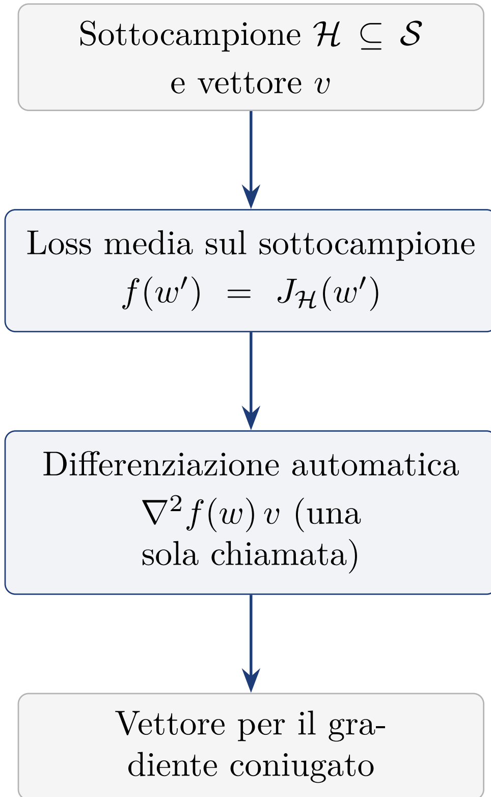
Figura 6.9. Prodotto Hessiano–vettore sul sottocampione: si definisce la loss media f sul batch Hessiano e se ne calcola \nabla^2 f(w) v in un’unica chiamata di differenziazione automatica, ottenendo lo stesso valore della media dei prodotti per-esempio.
