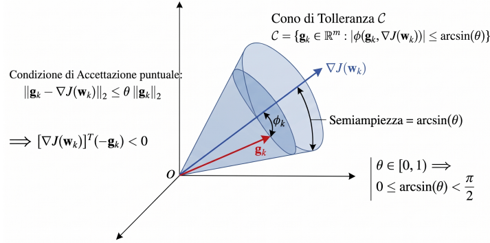
Figura 5.1. Rappresentazione geometrica della condizione di discesa: se il gradiente stimato g_k giace nel cono di tolleranza attorno al gradiente esatto \nabla J(w_k) , con errore \|e_k\| = \|g_k - \nabla J(w_k)\| \leq \theta \|g_k\| , allora -g_k è una direzione di discesa per J .
