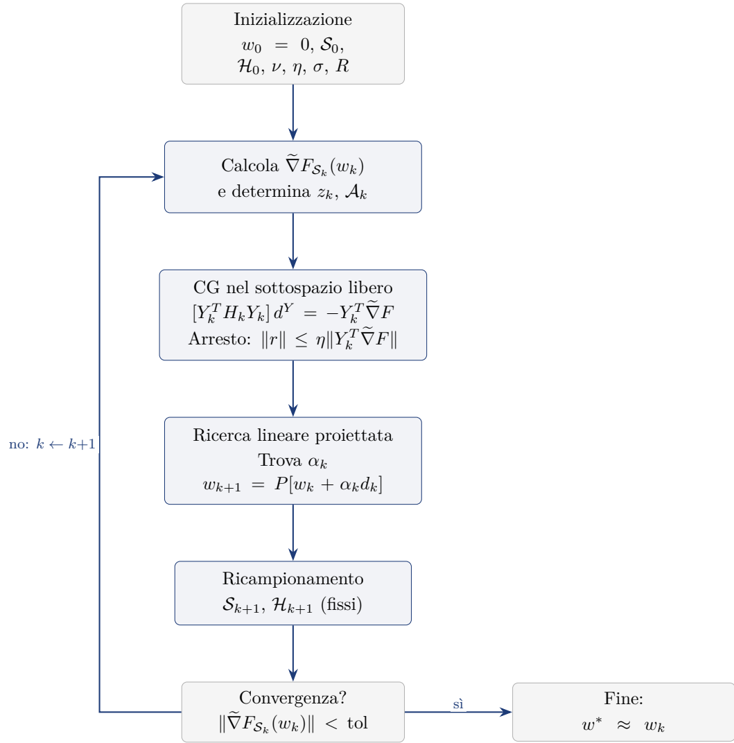
Figura 5.5. Schema del metodo Newton-CG per problemi con regolarizzazione L_1 : il gradiente generalizzato determina l'active set e la faccia ortante, il CG risolve il sistema ridotto sulle variabili libere e la ricerca lineare proiettata mantiene le variabili dell'active set a zero.
