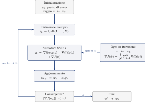
Figura D.1. Schema del metodo SVRG di Johnson e Zhang [9]: il punto di ancoraggio \bar{w} viene aggiornato ogni m iterazioni con il gradiente esatto \nabla J(\bar{w}) , e lo stimatore corregge il gradiente stocastico corrente con la differenza \nabla \ell(w_k; i_k) - \nabla \ell(\bar{w}; i_k) . Lo stimatore è non distorto, \mathbb{E}_{i_k}[g_k] = \nabla J(w_k) , e quando w_k è vicino a \bar{w} i due termini stocastici si elidono quasi del tutto, riducendo la varianza.
