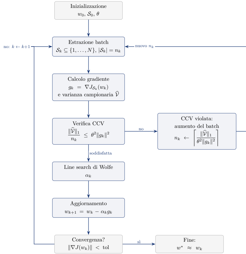
Figura 5.3. Schema dell'algoritmo con controllo della varianza campionaria (CCV): il flusso principale segue inizializzazione \rightarrow estrazione batch \rightarrow calcolo di gradiente e varianza \rightarrow verifica della CCV \rightarrow line search \rightarrow aggiornamento; quando la CCV è violata la dimensione del batch viene aumentata e si ripete l'estrazione.
