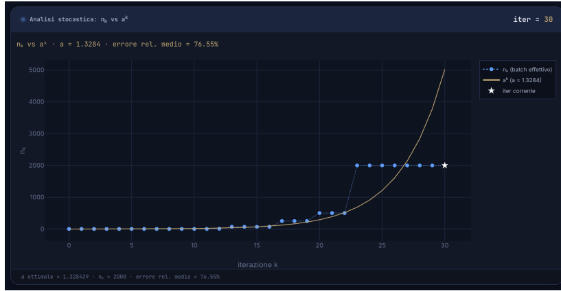
Figura 5.2. Andamento della dimensione del batch n_k in funzione dell'iterazione k per il metodo a campione dinamico (linea blu, con gradini in corrispondenza delle violazioni della CCV), confrontato con la funzione esponenziale a^k (curva oro). Il parametro a > 1 è stimato per minimi quadrati in scala logaritmica: minimizza \sum_k (\ln n_k - k \ln a)^2 , da cui \ln a = \frac{\sum_k k \ln n_k}{\sum_k k^2} . La crescita di n_k segue quindi una legge quasi geometrica n_k \approx a^k , concentrando la risorsa computazionale nelle iterazioni finali, dove il gradiente è piccolo e serve precisione.
