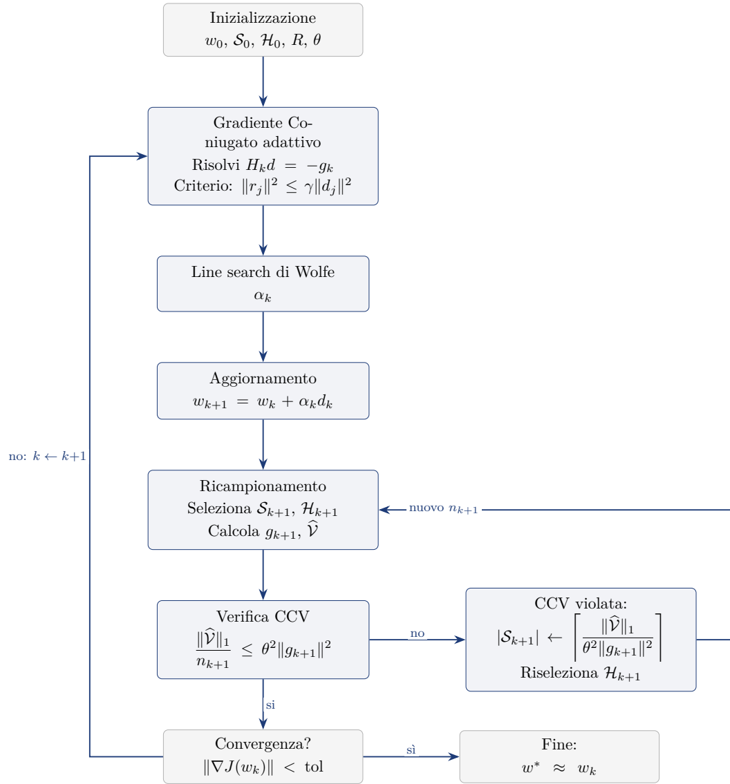
Figura 5.4. Schema del metodo Newton-CG con campionamento dinamico: ad ogni iterazione il gradiente coniugato risolve (in modo Hessian free) il sistema di Newton con un criterio di arresto adattivo; dopo l'aggiornamento e il ricampionamento, la CCV decide se aumentare la dimensione del batch.
