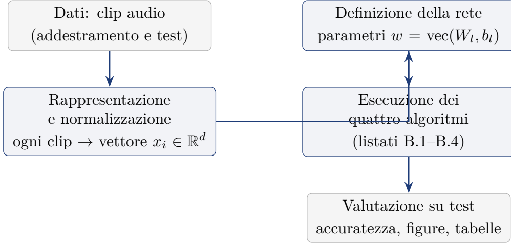
Figura 6.5. Pipeline sperimentale per la rete neurale: ogni clip audio è rappresentata da un vettore x_i di d descrittori che riassumono la distribuzione dell’energia del segnale nel tempo e in frequenza; i dati sono poi normalizzati e passati alla rete, su cui vengono eseguiti gli algoritmi dei listati B.1–B.4 con le funzioni batch vettorizzate.
