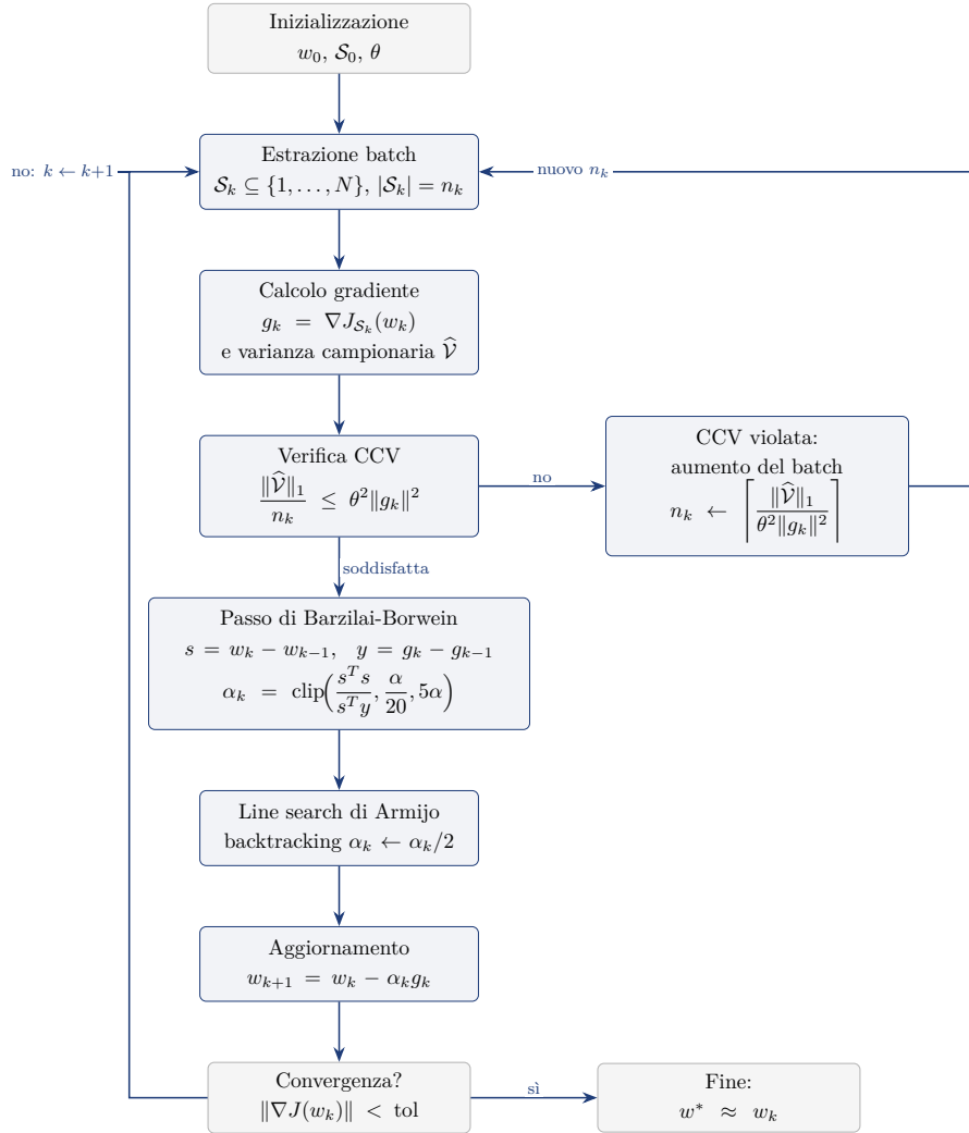
Figura E.1. Schema dell'algoritmo BB-CCV (gradiente a campione dinamico con passo di Barzilai–Borwein). Il flusso è quello del Dynamic GD (Figura 5.3): estrazione del batch \mathcal{S}_k , calcolo di gradiente e varianza campionaria \hat{\mathcal{V}} , verifica della CCV con eventuale aumento di n_k . La differenza è nel passo: per k > 0 si stima la curvatura di J usando solo i gradienti già calcolati, s = w_k - w_{k-1} e y = g_k - g_{k-1} , con la formula \alpha_k^{BB} = \frac{s^T s}{s^T y} di Barzilai–Borwein (per k = 0 , \alpha_0 = \alpha ); il passo è salvaguardato in [\alpha/20, 5\alpha] per la stabilità sui problemi non quadratici e rifinito da una line search di Armijo con backtracking. BB usa solo quantità già disponibili, quindi non richiede la Hessiana: negli esperimenti il metodo impiega 18 iterazioni medie (contro le 30 del GD) e sui problemi mal condizionati raggiunge precisioni 10^{-8} – 10^{-14} invece di 10^{-1} – 10^{-2} .
