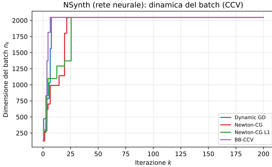
Figura 6.13: NSynth (rete neurale): dimensione del batch n_k scelta dal controllo CCV a ogni iterazione per i quattro metodi (tetto a 2048).
