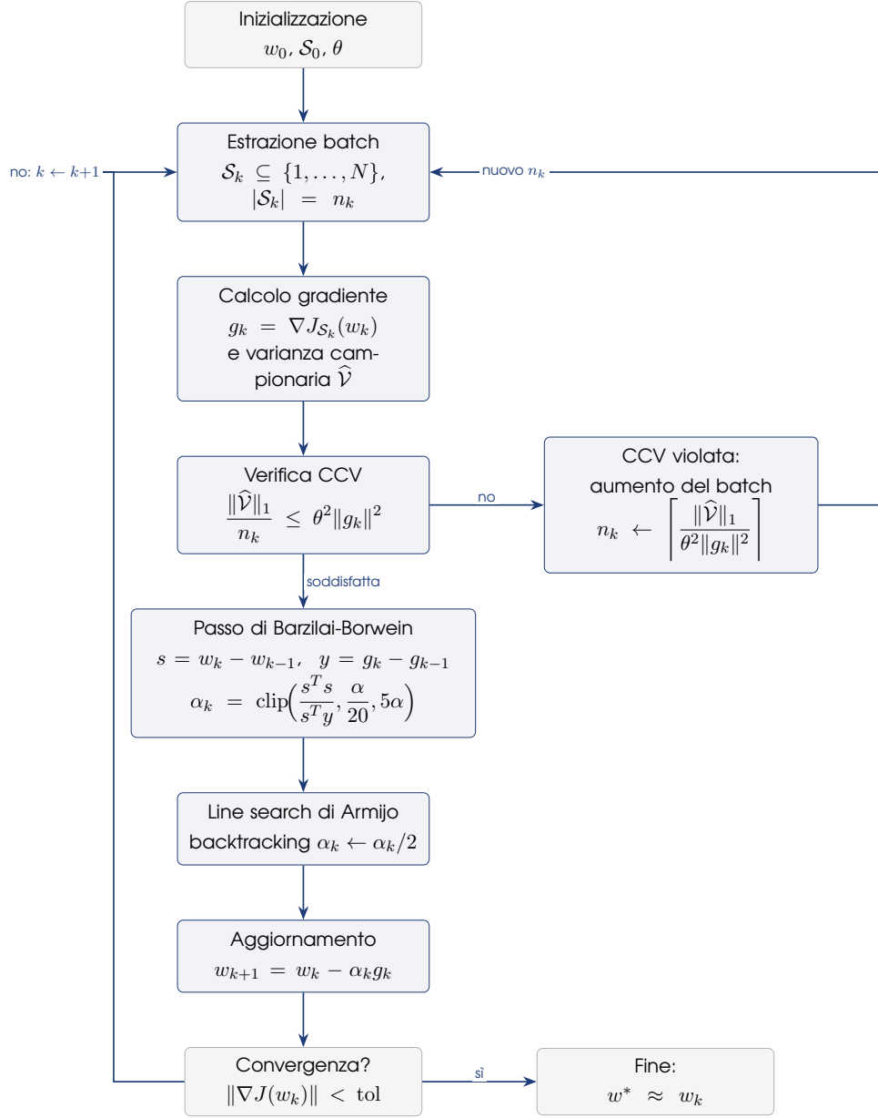
Figura E.1: Schema dell'algoritmo BB-CCV (gradiente a campione dinamico con passo di Barzilai-Borwein). Il flusso è quello del Dynamic GD (Figura 5.1): estrazione del batch S_k , calcolo di gradiente e varianza campionaria \hat{V} , verifica della CCV con eventuale aumento di n_k . La differenza è nel passo: per k > 0 si stima la curvatura di J usando solo i gradienti già calcolati, s = w_k - w_{k-1} e y = g_k - g_{k-1} , con la formula \alpha_k^{BB} = \frac{s^T s}{s^T y} di Barzilai-Borwein (per k = 0 , \alpha_0 = \alpha ); il passo è salvaguardato in [\alpha/20, 5\alpha] per la stabilità sui problemi non quadratici e rifinito da una line search di Armijo con backtracking. BB usa solo quantità già disponibili, quindi non richiede la Hessiana: negli esperimenti il metodo impiega 18 iterazioni medie (contro le 30 del GD) e sui problemi mal condizionati raggiunge precisioni 10^{-8} – 10^{-14} invece di 10^{-1} – 10^{-2} .
