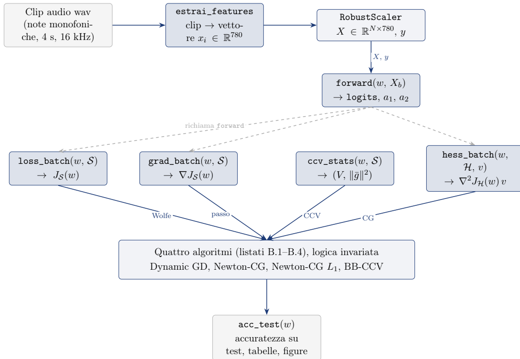
Figura 6.3: Mappa delle funzioni dell'implementazione vettorizzata. Dalle clip si estraggono i vettori x_i (Figura 6.4), normalizzati nella matrice X ; forward calcola le attivazioni della rete e le quattro funzioni che la richiamano forniscono agli algoritmi dei listati B.1–B.4 proprio gli oggetti che essi richiedono: la loss per la line search di Wolfe, il gradiente per il passo, la varianza per la verifica CCV e il prodotto Hessiano–vettore per il gradiente coniugato; acc_test valuta infine la soluzione sul test. Freccie continue: flusso dei dati; frecce tratteggiate: chiamate tra funzioni.
