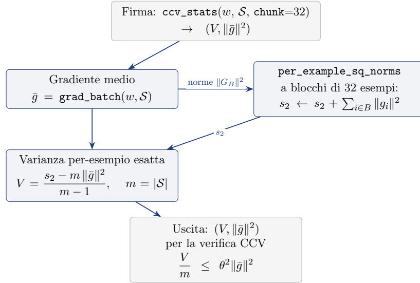
Figura 6.8: Funzione ccv_stats : gradiente medio dal grad_batch , somma dei quadrati delle norme per-esempio calcolata a blocchi di 32 esempi (per non materializzare la matrice n_k \times D ) e combinazione nella formula esatta della varianza campionaria; l'uscita alimenta la verifica CCV del listato B.1.
