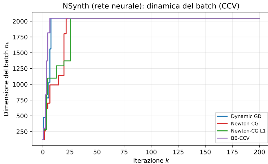
Figura 6.11: NSynth (rete neurale): dimensione del batch n_k scelta dal controllo CCV a ogni iterazione per i quattro metodi (tetto a 2048).
