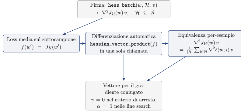
Figura 6.9: Funzione hess_batch : il prodotto Hessiano–vettore sul sottocampione \mathcal{H} è calcolato definendo la loss media f e chiamando hessian_vector_product una sola volta; il valore coincide con la media dei prodotti per-esempio.
