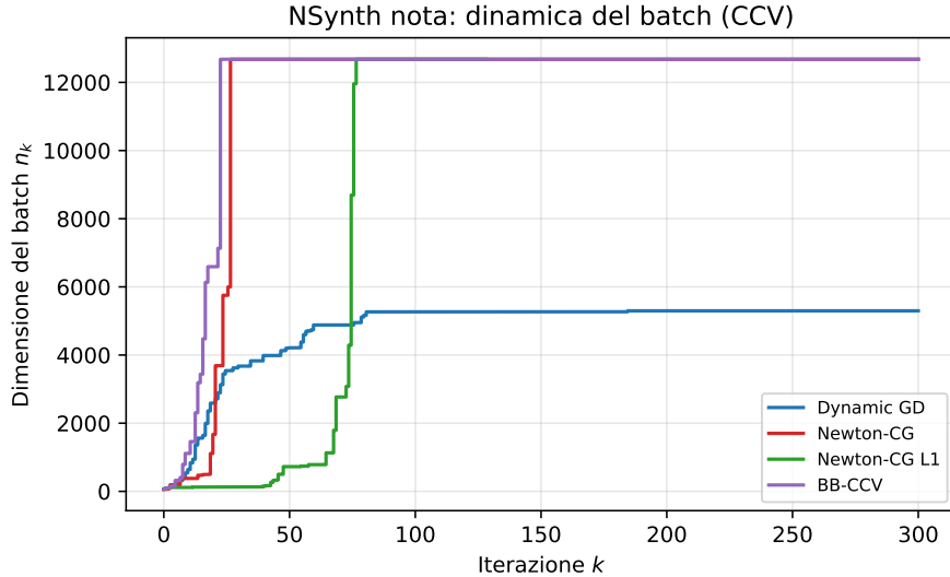
Figura 6.2: Dimensione del batch n_k per il riconoscimento della nota: anche su questo compito la CCV aumenta il campione man mano che il gradiente si riduce.
