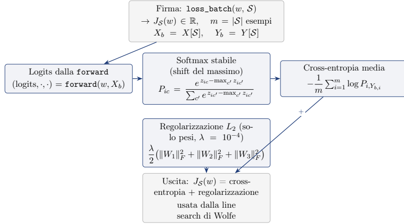
Figura 6.6: Funzione loss_batch : logits dalla forward , softmax stabile, cross-entropia media sul batch e regolarizzazione L_2 sui pesi; l'uscita è la somma dei due contributi.
