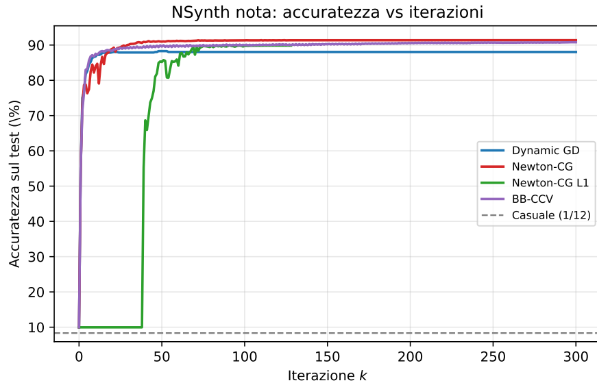
Figura 6.1: Accuratezza sul test NSynth per il riconoscimento della nota in funzione delle iterazioni k . La linea tratteggiata indica la predizione casuale ( 1/12 \approx 8.3\% ).
