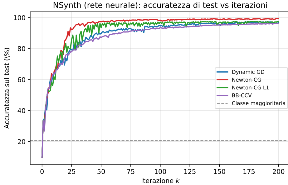
Figura 6.10: NSynth (rete neurale): accuratezza sul test set in funzione delle iterazioni per i quattro metodi; la linea tratteggiata indica la frequenza della classe maggioritaria (20.8%).
