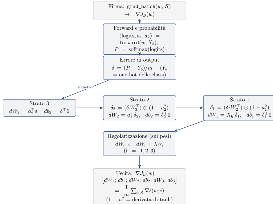
Figura 6.7: Funzione grad_batch : retropropagazione vettorizzata. L'errore \delta tra probabilità e one-hot è propagato all'indietro con la derivata di \tanh ( 1 - a^2 ); a ogni matrice dei pesi si somma \lambda W_l . Il risultato coincide con la media dei gradienti per-esempio del listato B.1.
