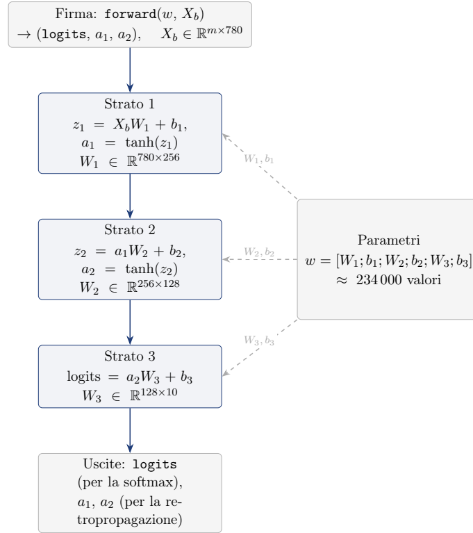
Figura 6.5: Funzione forward (architettura della rete): tre trasformazioni affini intervallate dall'attivazione \tanh , con le dimensioni delle matrici; w è l'intero vettore dei parametri, da cui ogni strato legge i propri pesi W_l e bias b_l . I logits sono le uscite grezze dell'ultimo strato.
