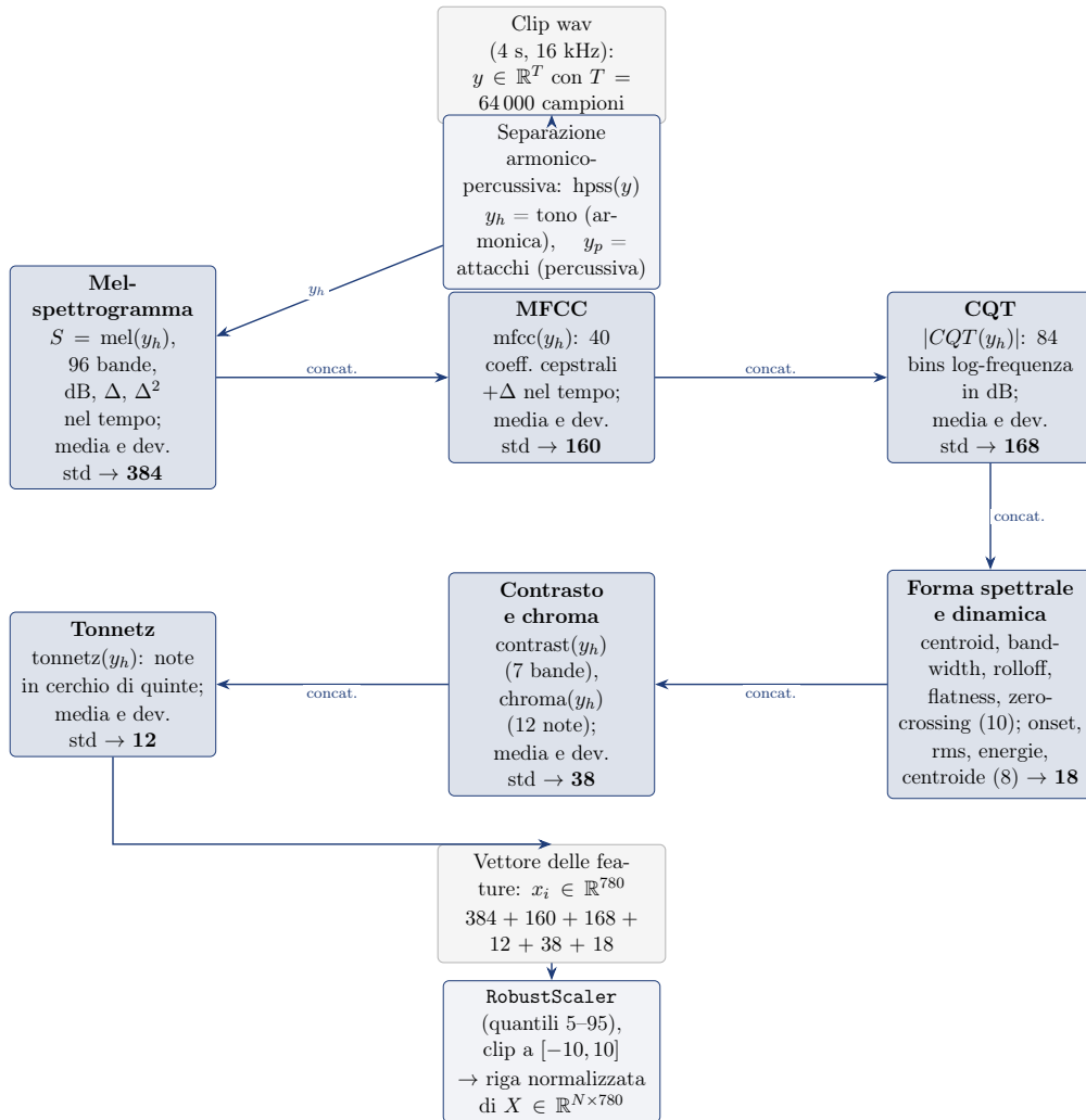
Figura 6.4: estrai_features : da clip audio a vettore di feature. Il segnale y è separato in armonica ( y_h ) e percussiva ( y_p ); sei famiglie di descrittori calcolati su y_h (tonnetz, spettrale e dinamica anche su y ) producono medie e deviazioni standard nel tempo, concatenate nel vettore x_i \in \mathbb{R}^{780} (le cifre indicano le dimensioni di ogni blocco); infine RobustScaler normalizza le colonne sui quantili 5–95 e i valori sono limitati a [-10, 10] . Le frecce etichettate concat. indicano che i blocchi, calcolati indipendentemente, sono concatenati nell'ordine mostrato.
