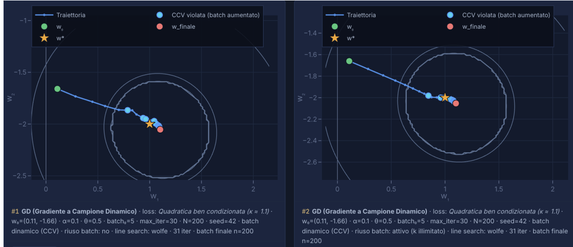
Figura 6.1: Traiettorie di Dynamic GD sul problema quadratico ben condizionato ( \kappa \approx 1.1 ) dal pannello Traiettorie 2D dell'applicazione: (in alto) ricampionamento a ogni iterazione; (in basso) riuso illimitato dello stesso mini-batch ( M = \infty ). Punto iniziale w_0 = (0.11, -1.66) , \alpha = 0.1 , \theta = 0.5 , n_0 = 5 , 30 iterazioni, seed 42; i punti marcati indicano le iterazioni in cui la condizione CCV risulta violata (batch aumentato).
