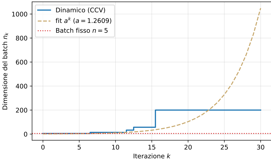
Evoluzione dinamica della dimensione del batch (CCV)
