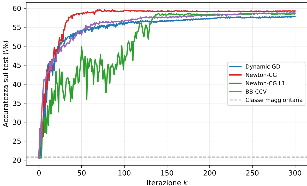
NSynth: accuratezza di test vs iterazioni
