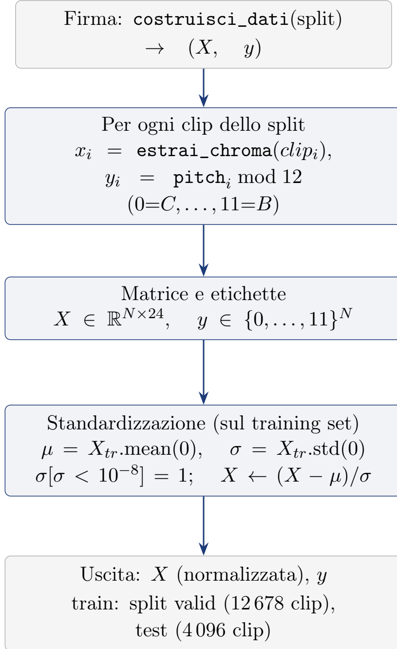
Figura 6.3: Funzione costruisci_dati : costruisce la matrice delle features e le etichette della pitch class per uno split, poi le normalizza con media e deviazione standard calcolate sul solo training set (le stesse statistiche sono applicate a test).
