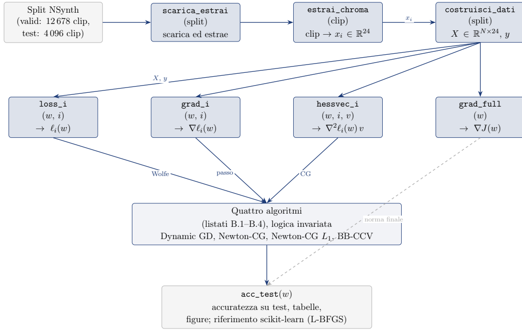
Figura 6.1: Mappa delle funzioni del notebook nsynth_note_reproduzione . Dalle clip di uno split si estraggono i vettori x_i (Figura 6.2), raccolti in X con le etichette delle note da costruisci_dati ; le quattro funzioni del nucleo forniscono agli algoritmi dei listati B.1–B.4 proprio gli oggetti che essi richiedono: la loss per la line search di Wolfe, il gradiente per il passo, il prodotto Hessiano–vettore per il gradiente coniugato; grad_full e acc_test servono alle metriche di valutazione. Freccie continue: flusso dei dati; frecce tratteggiate: chiamate tra funzioni.
