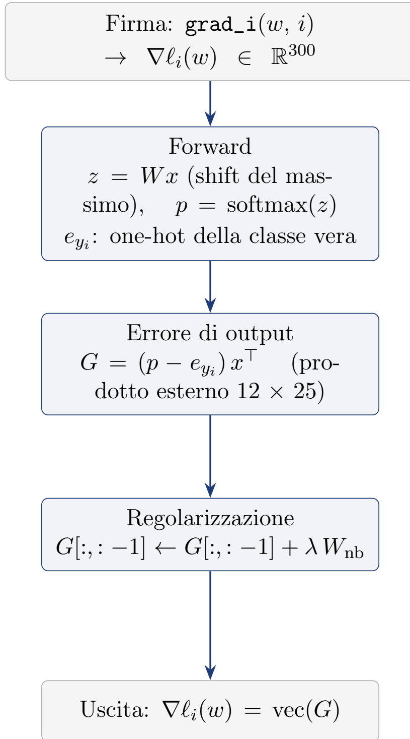
Figura 6.5: Funzione grad_i : gradiente per-esempio della regressione logistica. L'errore p - e_{y_i} tra le probabilità e la codifica one-hot della classe vera, esteriorizzato con l'input x , dà la matrice 12 \times 25 ; la colonna del bias (l'ultima) non riceve regolarizzazione.
