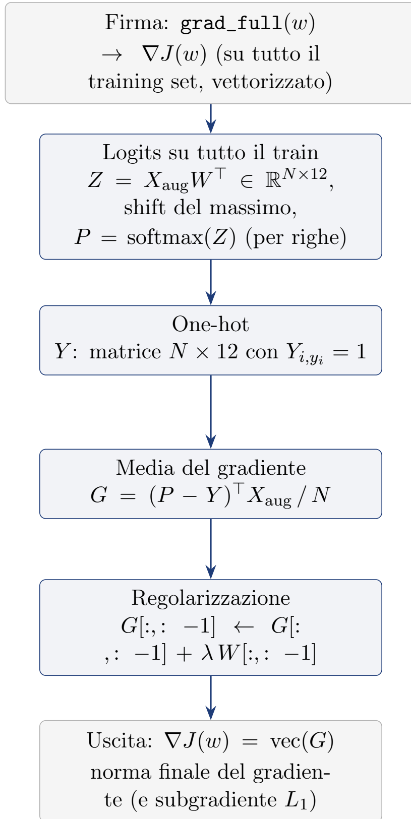
Figura 6.7: Funzione grad_full : gradiente di J su tutto il training set in forma matriciale. Le probabilità di tutte le N clip sono calcolate in un unico prodotto; la media degli errori (P - Y) pesati con le features dà il gradiente, usato per la norma finale e per il subgradiente del metodo L_1 .
