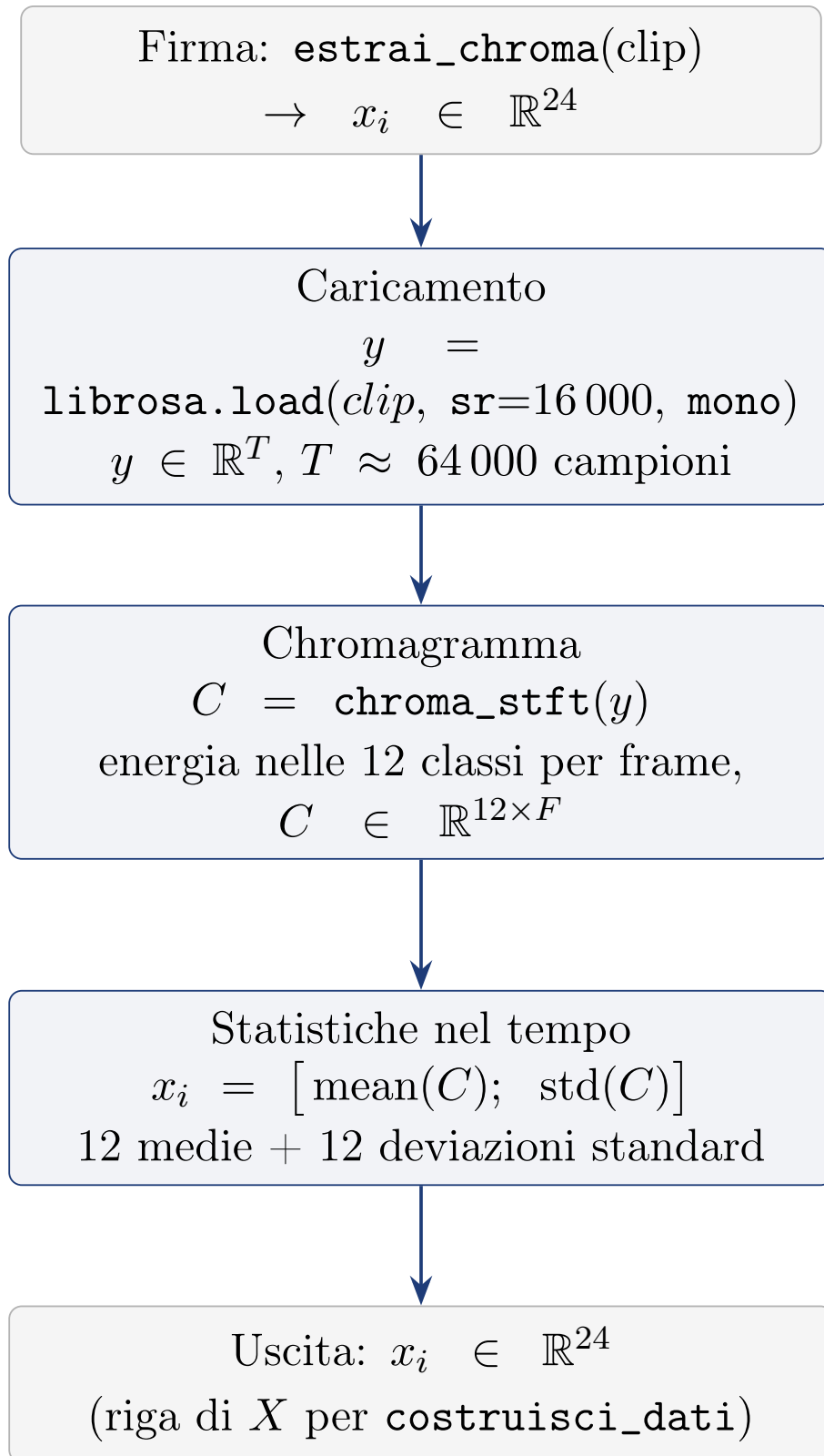
Figura 6.2: Funzione estrai_chroma : da clip audio a vettore di 24 statistiche cromatiche. Il chromagramma C misura l'energia in ciascuna delle 12 classi di altezza in ogni frame temporale; media e deviazione standard nel tempo producono il vettore x_i .
