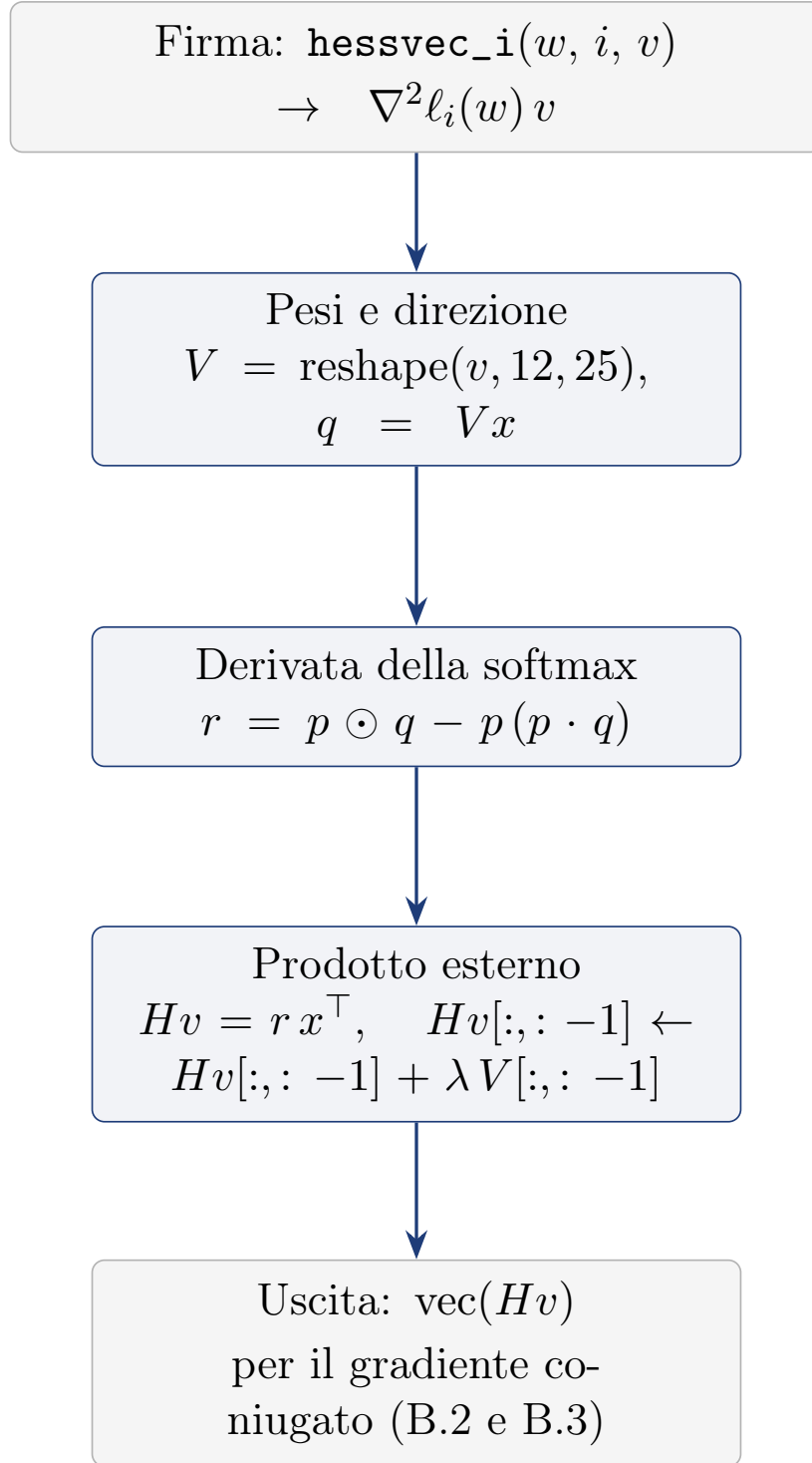
Figura 6.6: Funzione hessvec_i : prodotto Hessiano–vettore per-esempio. L’Hessiana della regressione logistica applicata a v richiede la derivata della softmax lungo la direzione q = Vx ; la regolarizzazione L_2 contribuisce solo sulle colonne dei pesi.
