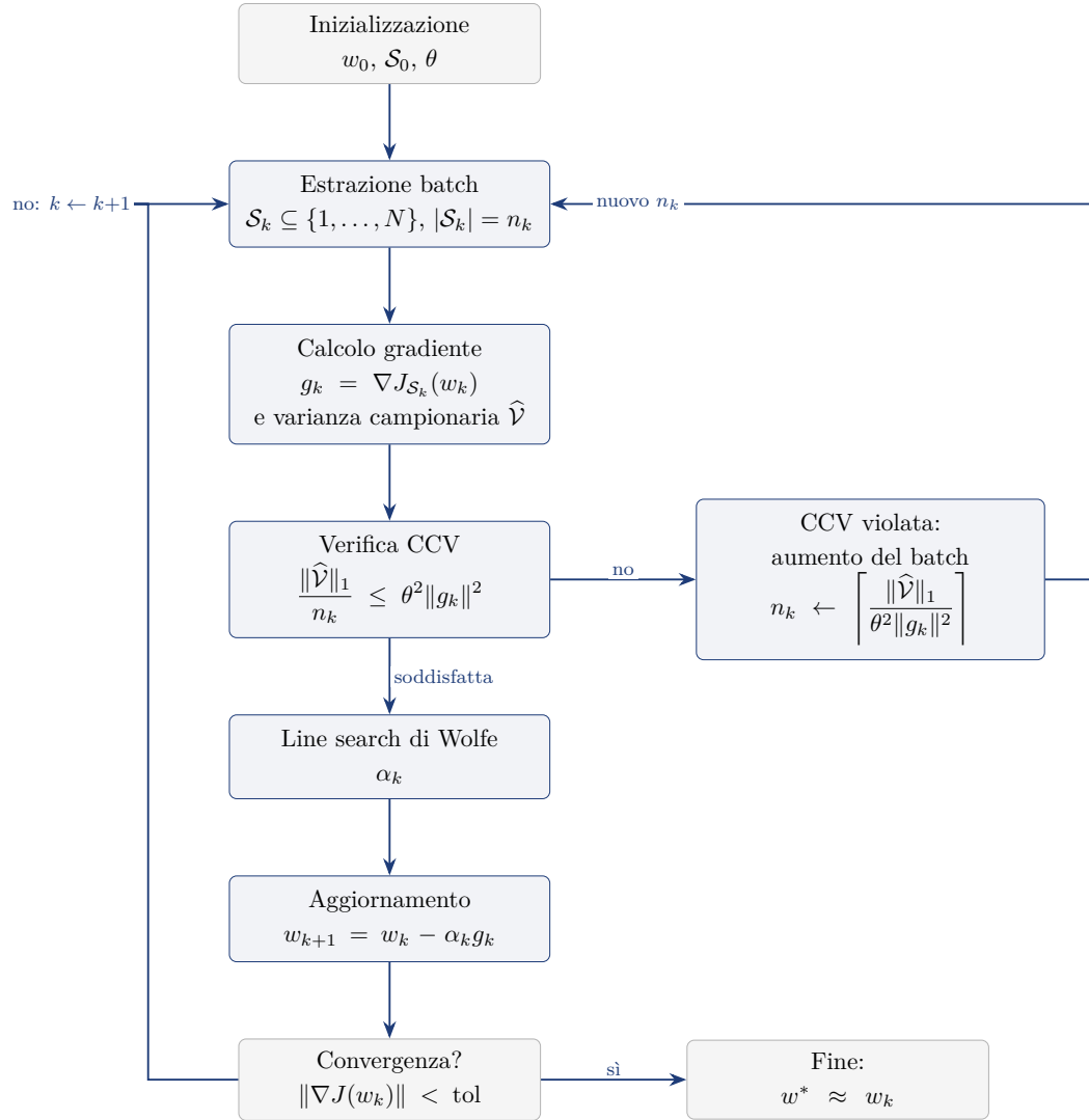
Figura 5.1. Schema dell'algoritmo con controllo della varianza campionaria (CCV): il flusso principale segue inizializzazione \rightarrow estrazione batch \rightarrow calcolo di gradiente e varianza \rightarrow verifica della CCV \rightarrow line search \rightarrow aggiornamento; quando la CCV è violata la dimensione del batch viene aumentata e si ripete l'estrazione.
