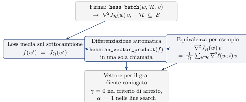
Figura 6.11: Funzione hess_batch : il prodotto Hessiano–vettore sul sottocampione \mathcal{H} è calcolato definendo la loss media f e chiamando hessian_vector_product una sola volta; il valore coincide con la media dei prodotti per-esempio.
