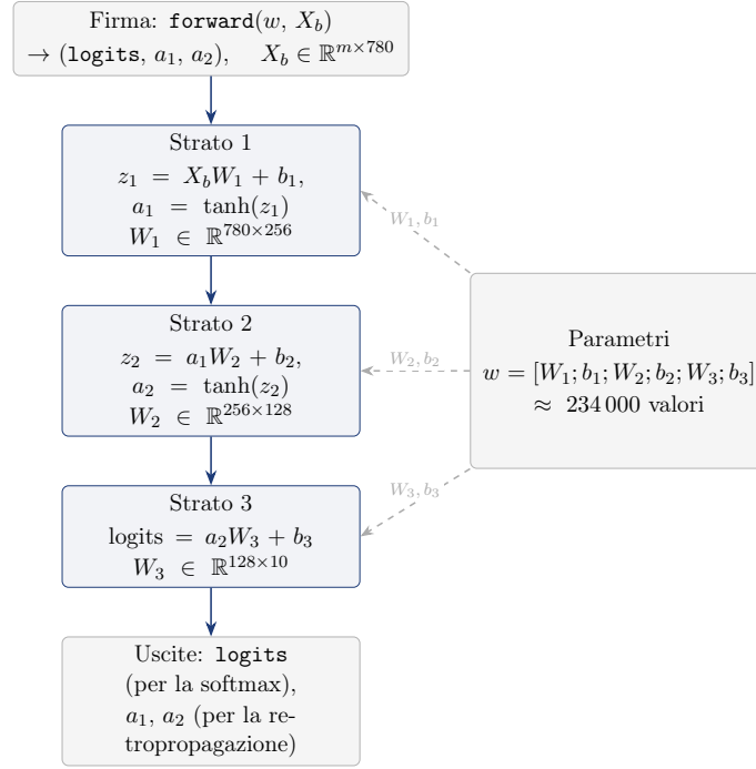
Figura 6.7: Funzione forward (architettura della rete): tre trasformazioni affini intervallate dall’attivazione tanh, con le dimensioni delle matrici; w è l’intero vettore dei parametri, da cui ogni strato legge i propri pesi W_l e bias b_l . I logits sono le uscite grezze dell’ultimo strato.
