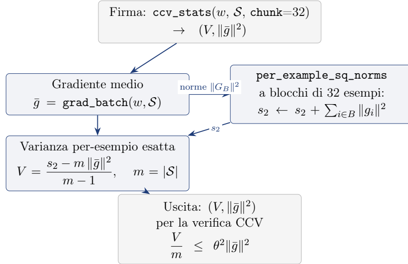
Figura 6.10: Funzione ccv_stats : gradiente medio dal grad_batch , somma dei quadrati delle norme per-esempio calcolata a blocchi di 32 esempi (per non materializzare la matrice n_k \times D ) e combinazione nella formula esatta della varianza campionaria; l’uscita alimenta la verifica CCV del listato B.1.
