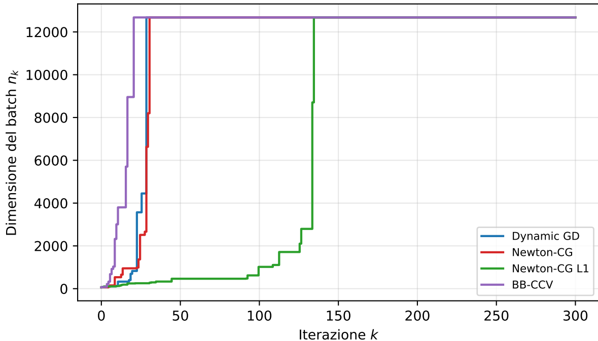
NSynth: dinamica del batch (CCV)
