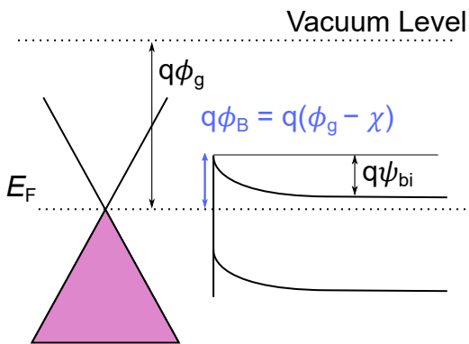
Thermal Equilibrium (zero bias)
