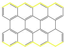
zigzag
