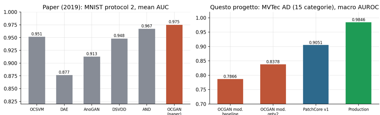
Figura 10 — I risultati del paper sui suoi dataset (sinistra) e i nostri su MVTec AD (destra). I numeri non sono direttamente confrontabili: dataset, protocolli ed epoche di letteratura diverse.
