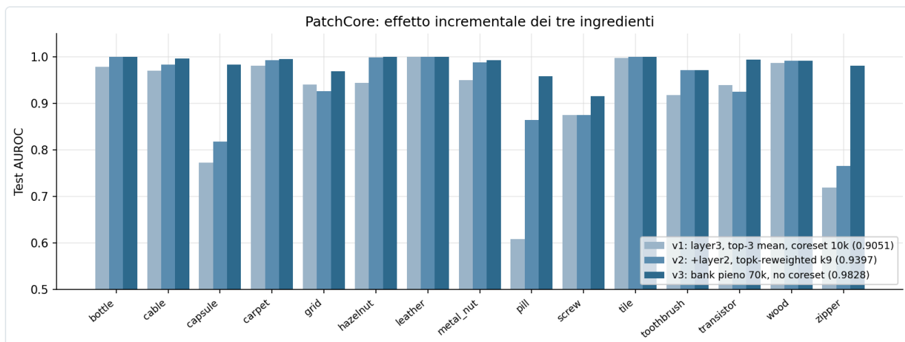
Figura 7 — Le tre versioni di PatchCore per categoria: ogni ingrediente recupera categorie diverse.
