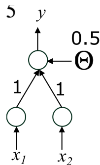
Figura 109: Rete neurale per "OR"
