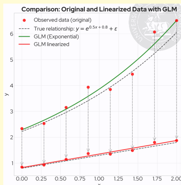
Figura 66: Confronto: originale e linearizzato con GLM
