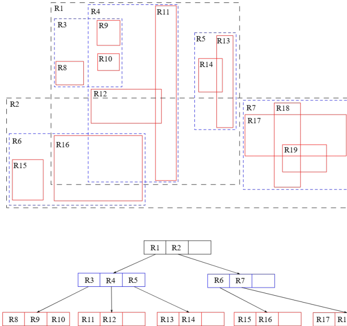
Figura 74: Esempio di R-tree: gerarchia dei Minimum Bounding Rectangles
