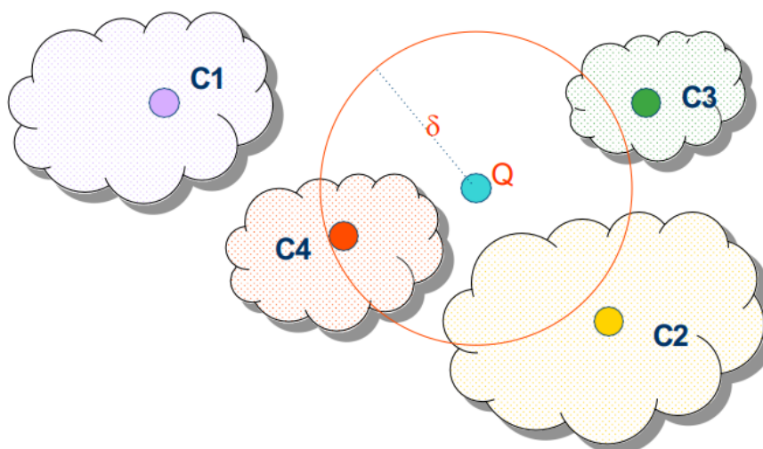
Figura 85: Query di range in uno spazio con cluster
