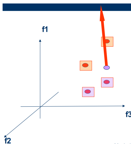
Figura 108: Applicazione della direzione di spostamento alla query Q
