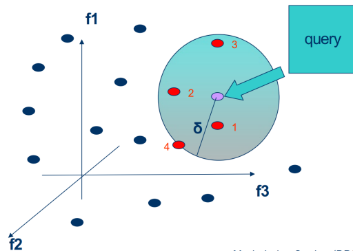
Figura 105: Query di range iniziale
