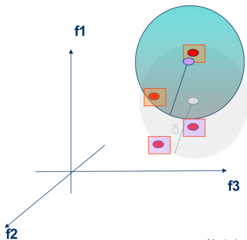
Figura 109: Nuova query Q' centrata nel cluster ottimale
