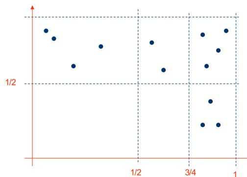
Figura 64: Esempio di file a griglia
