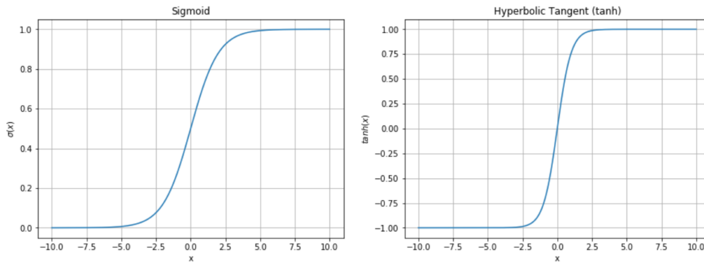
Figura 97: Funzione di attivazione Sigmoid e Hyperbolic Tangent
