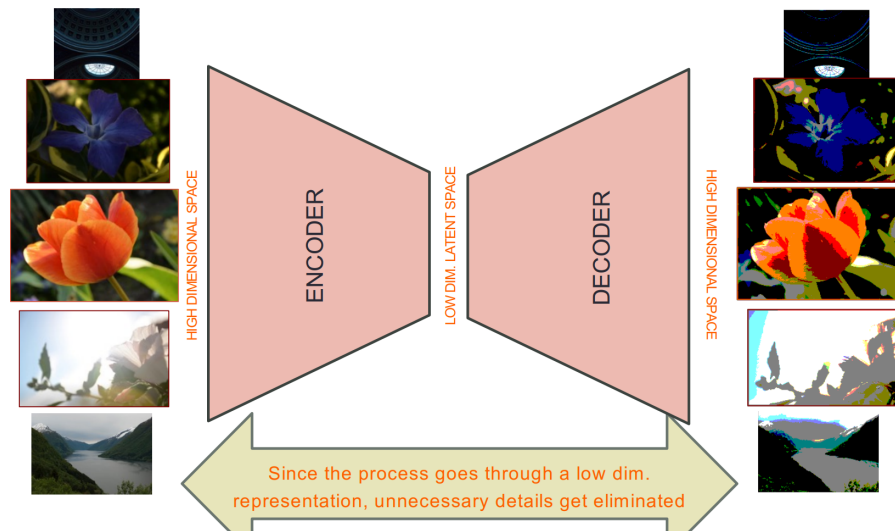
Figura 94: Architettura Encoder/Decoder: compressione nello spazio latente e successiva ricostruzione
