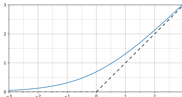
Figura 96: Funzione di attivazione SoftPlus
