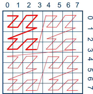
Figura 61: Esempio di curva Z-order e della sua struttura frattale
