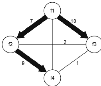
Figura 93: Albero di copertura massima (Maximum Spanning Tree)
