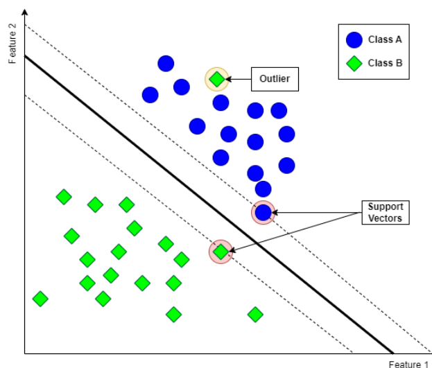
Figura 90: Esempio di Support Vector Machine in uno spazio bidimensionale
