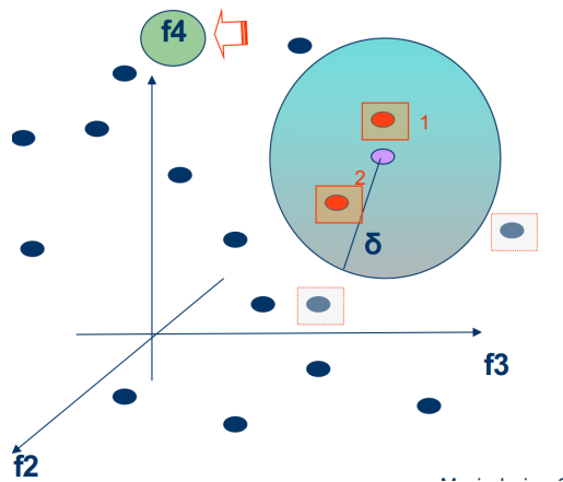
Figura 102: Query modificata aggiungendo e rimuovendo feature
