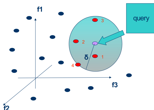
Figura 98: Query di range iniziale
