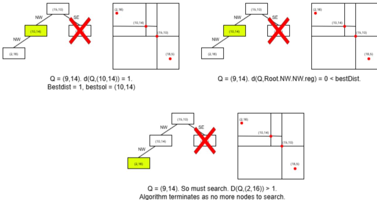
Figura 69: Esempio di ricerca NN nello spazio partizionato
