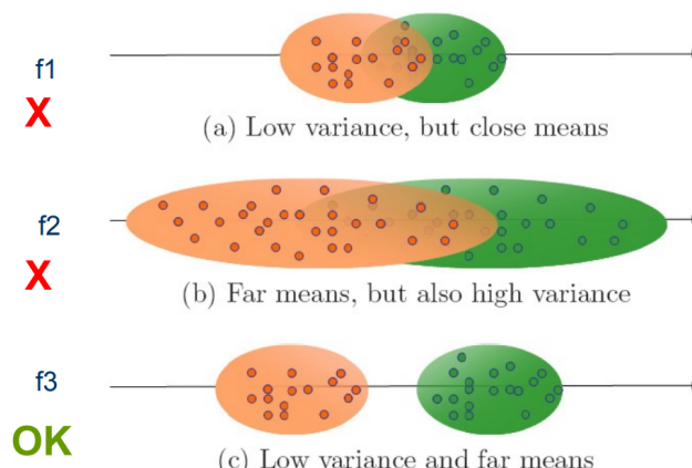
Figura 91: L'FSR premia le feature che presentano una grande distanza tra le medie delle classi (alta separazione) e una bassa varianza (alta compattezza).
