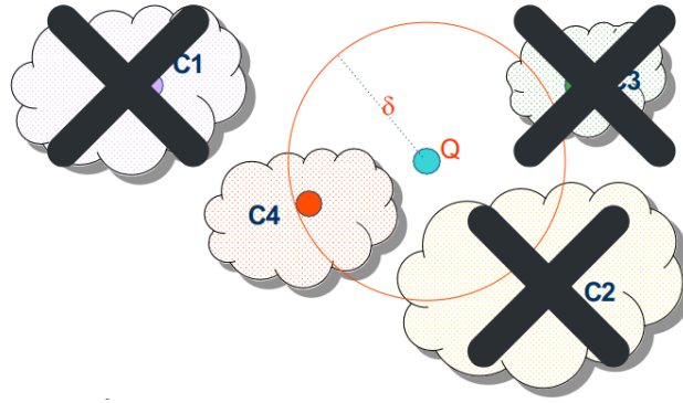
Figura 86: Falsi negativi (Misses) in una query di range
