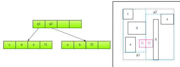
Figura 75: Esempio di R+ tree con oggetti clippati per evitare sovrapposizioni
