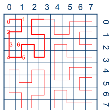
Figura 63: Esempio di curva di Peano-Hilbert e dei suoi passaggi adiacenti
