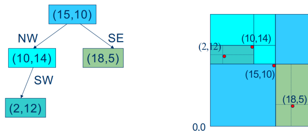
Figura 68: Esempio di quadtree di punti: fase finale
