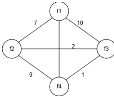
Figura 92: Grafo di dipendenza iniziale (completo)
