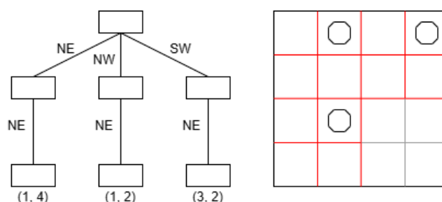
Figura 73: Esempio di inserimento finale: la griglia è regolare
