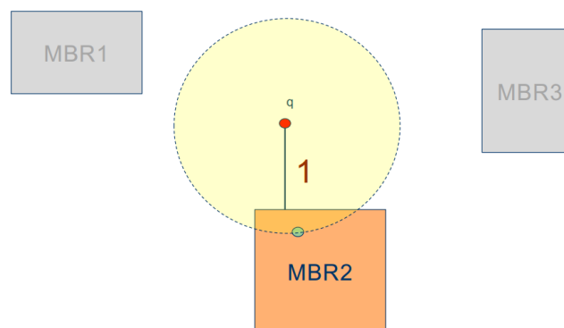
Figura 76: Esempio di calcolo minDist
