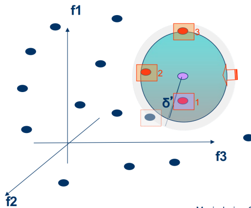
Figura 100: Query di range modificando il raggio
