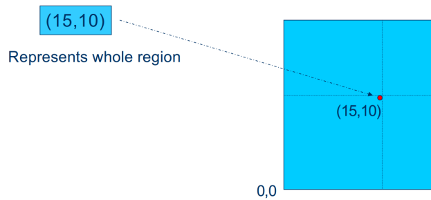
Figura 66: Esempio di quadtree di punti: partizionamento iniziale dalla radice
