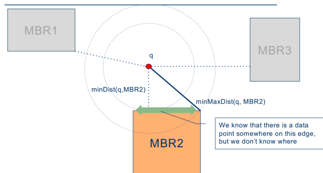
Figura 78: Esempio di minMaxDist fase finale
