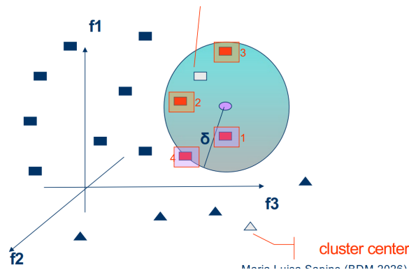
Figura 104: Riorganizzazione dello spazio tramite clustering
