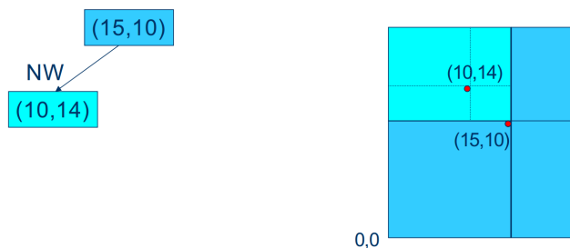
Figura 67: Esempio di quadtree di punti: inserimento di un nuovo punto
