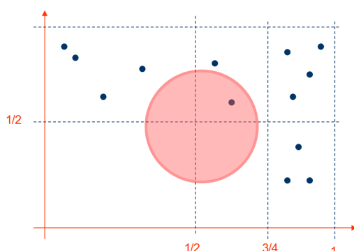
Figura 65: Esempio di file a griglia con accesso a pagine vuote
