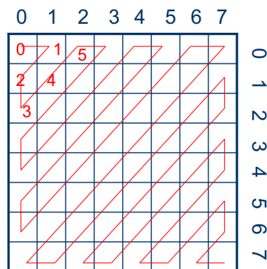
Figura 60: Esempio di ordine diagonale di Cantor
