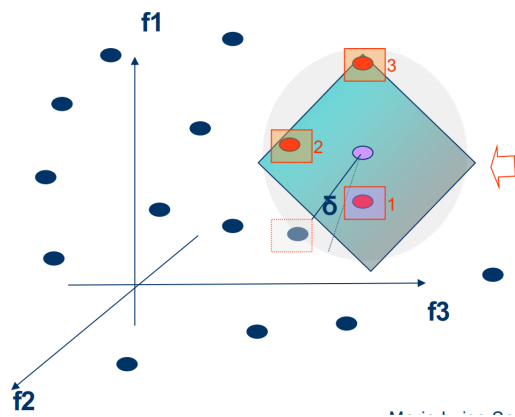
Figura 103: Query di range modificando la metrica di distanza
