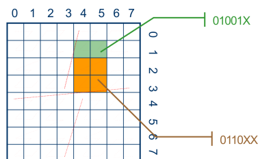
Figura 62: Esempio di raggruppamento di punti vicini (range) tramite prefissi binari nella curva Z-order
