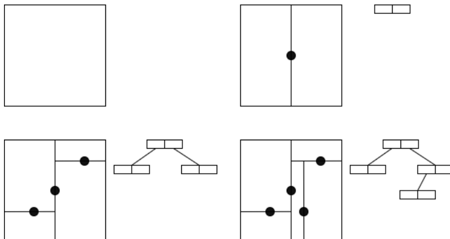
Figura 71: Esempio di inserimento e suddivisione alternata in un KD tree
