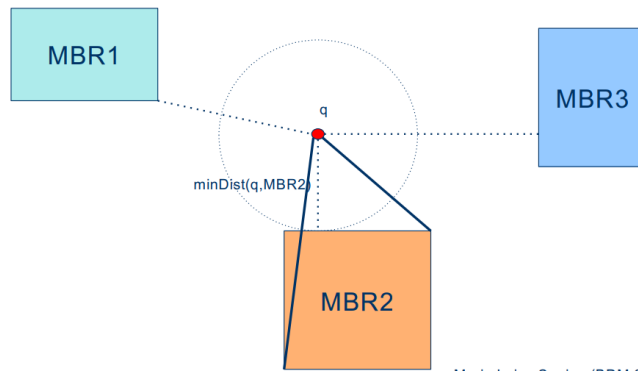
Figura 77: Esempio di minMaxDist fase iniziale
