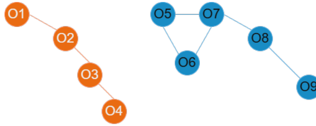
Figura 87: Esempio di clusterizzazione con componenti connesse (Effetto catena)
