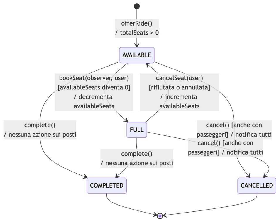
Figura 11 — State Diagram di Ride
