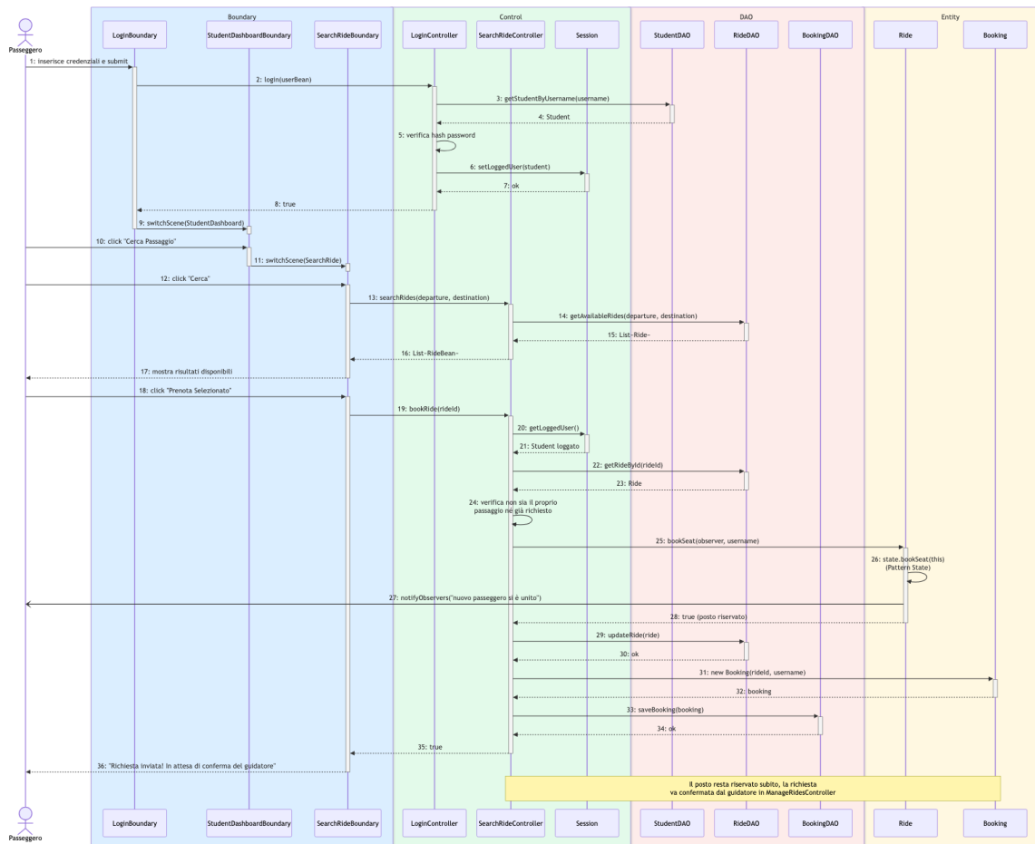
Figura 10 — Sequence Diagram del flusso login → ricerca → richiesta di prenotazione
