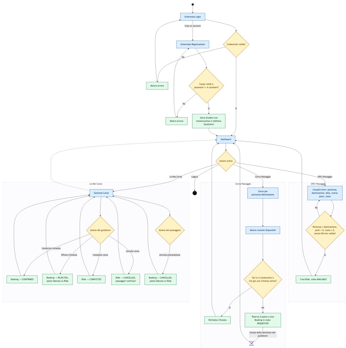
Figura 9 — Diagramma di attività del flusso applicativo principale
