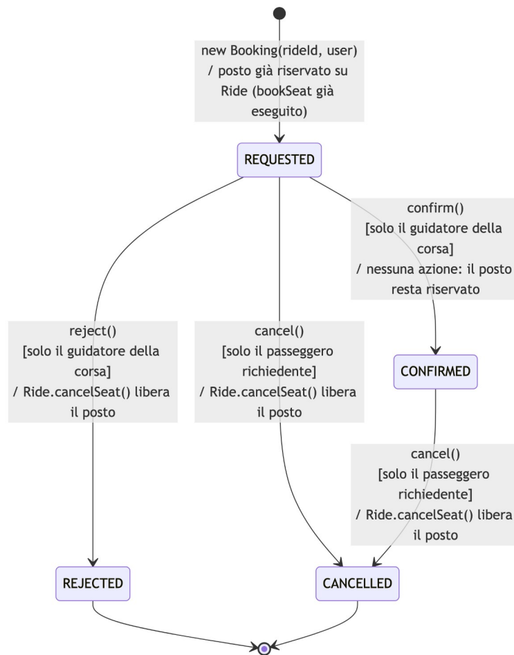
Figura 12 — State Diagram di Booking
