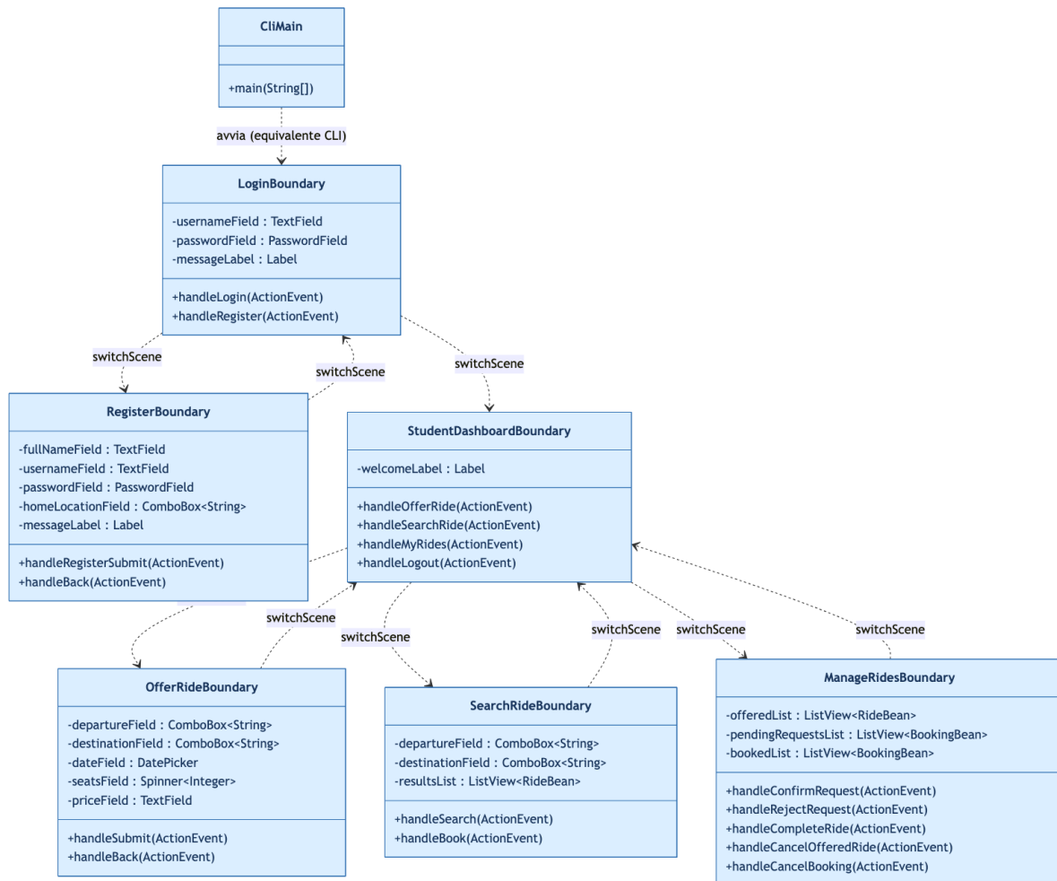
Figura 2 — Diagramma delle classi Boundary
