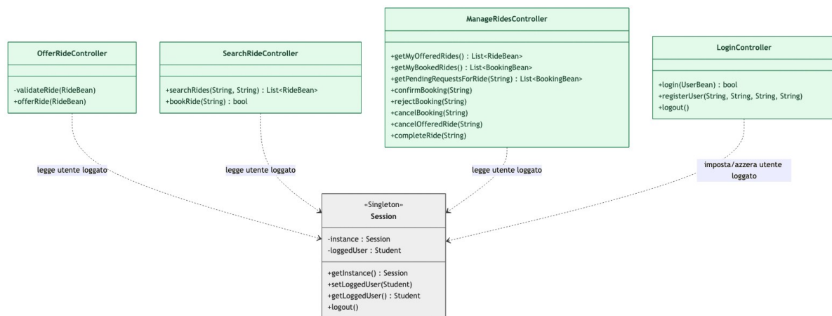
Figura 3 — Diagramma delle classi Control
