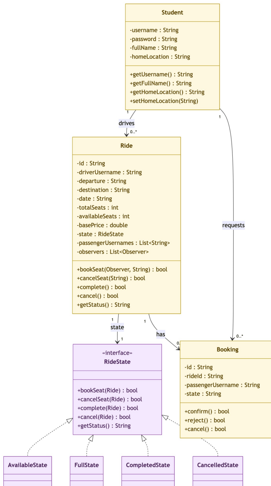
Figura 4 — Diagramma delle classi Entity
