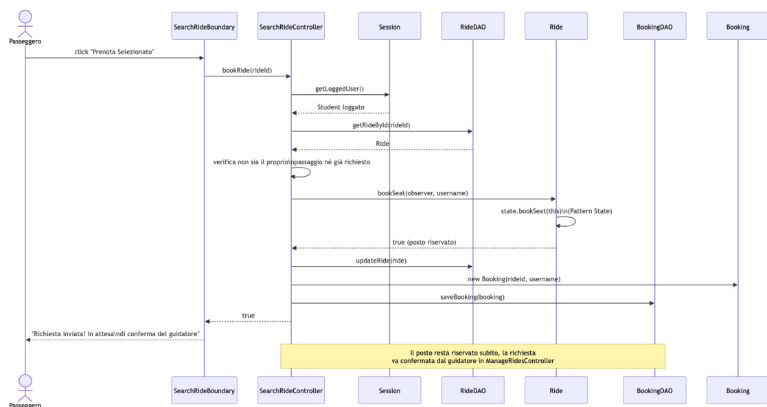
Figura 12 — Sequence Diagram del caso d'uso 'Richiedi Prenotazione'
