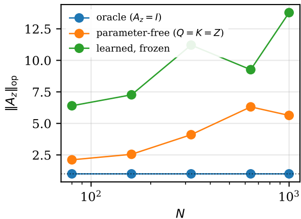
(d) operator op-norm grows, yet (a)-(c) hold
