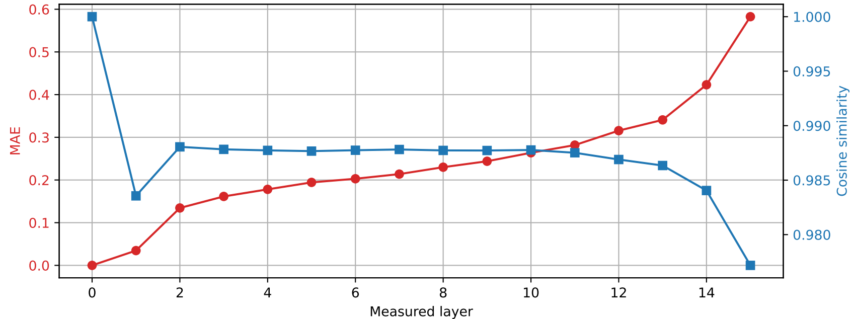
Llama-3.2-1B | Prompt 0 Spared layer 3 | Hybrid vs unquantized
