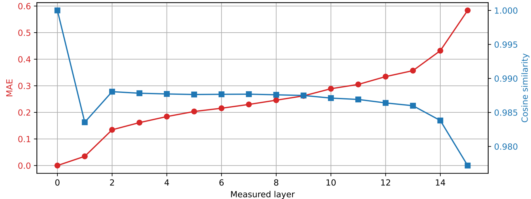
Llama-3.2-1B | Prompt 0 Spared layer 9 | Hybrid vs unquantized
