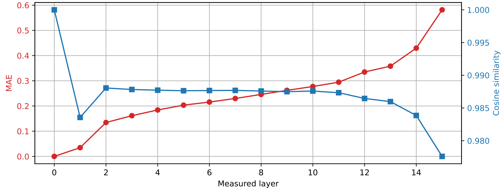
Llama-3.2-1B | Prompt 0 Spared layer 11 | Hybrid vs unquantized
