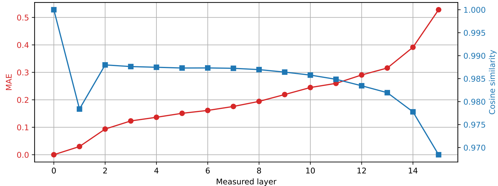
Llama-3.2-1B | Prompt 1 Spared layer 3 | Hybrid vs unquantized
