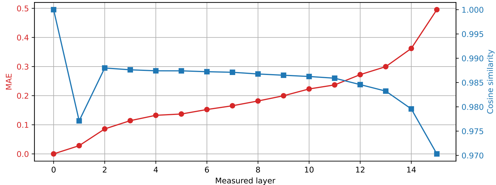
Llama-3.2-1B | Prompt 2 Spared layer 4 | Hybrid vs unquantized
