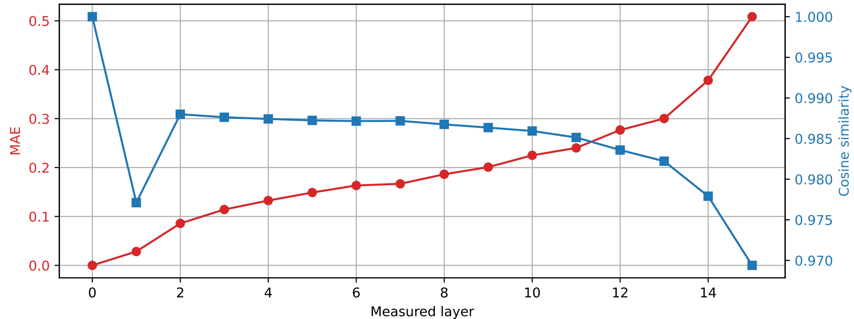
Llama-3.2-1B | Prompt 2 Spared layer 6 | Hybrid vs unquantized
