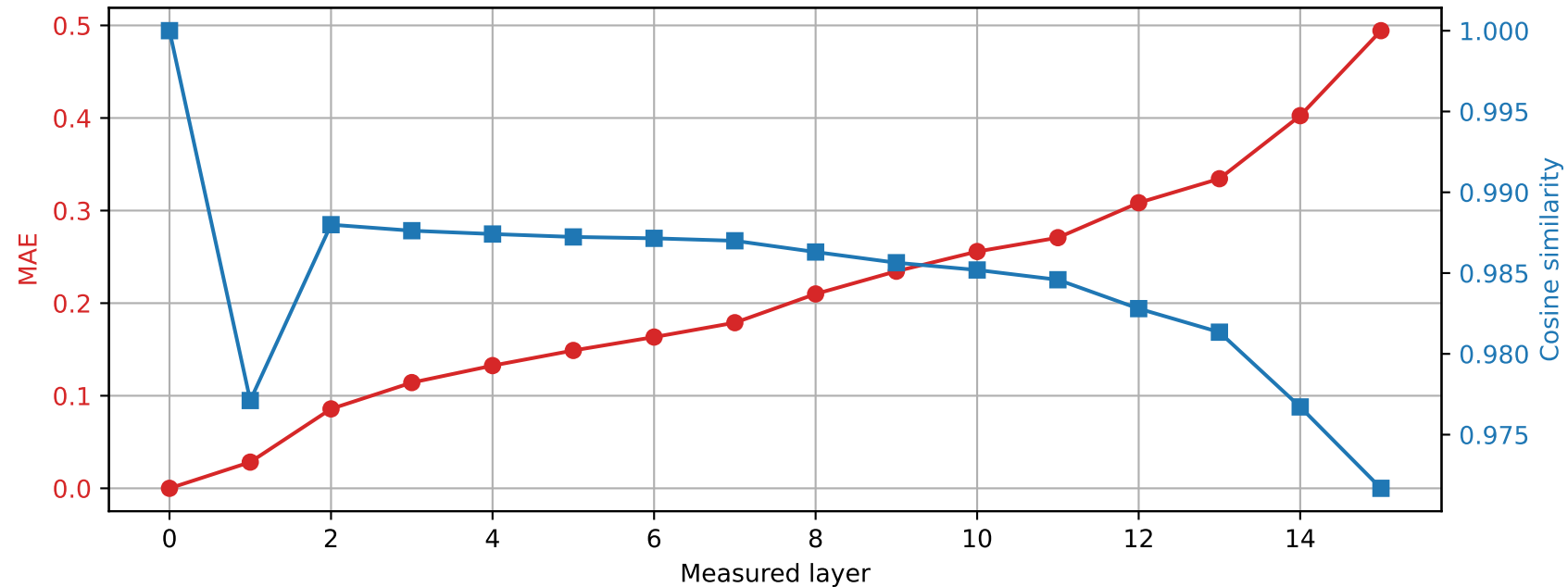
Llama-3.2-1B | Prompt 2 Spared layer 14 | Hybrid vs unquantized
