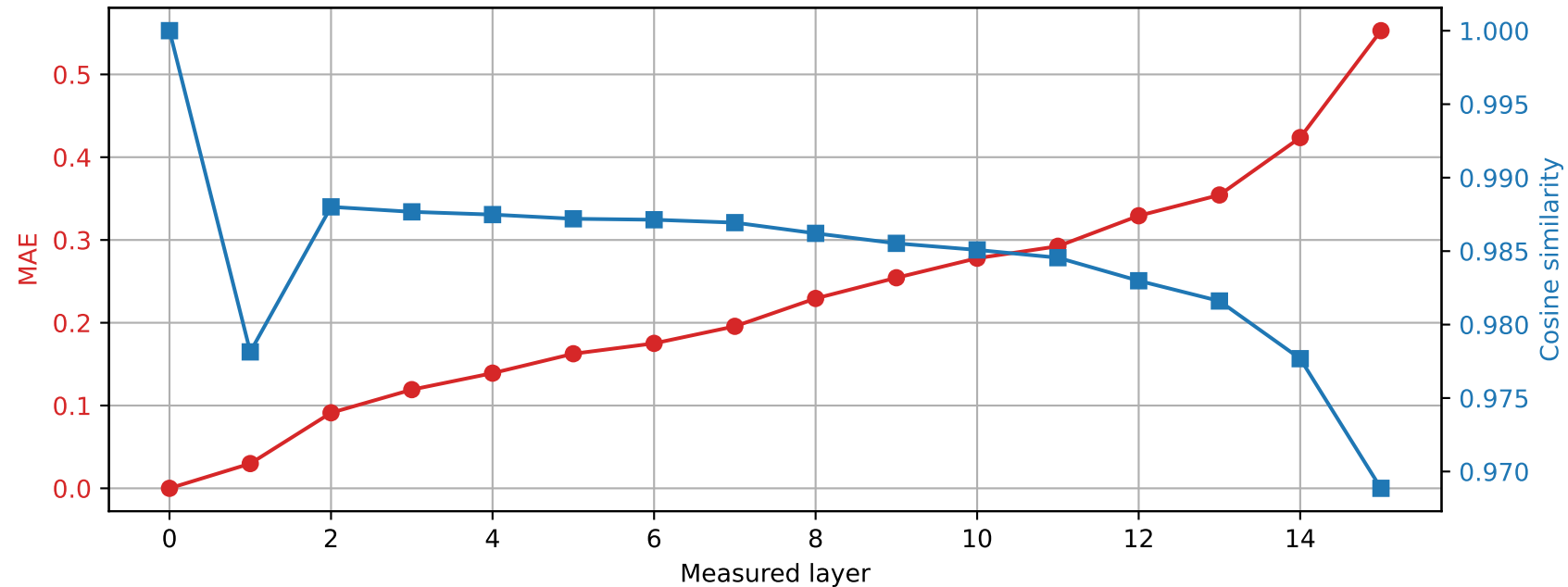
Llama-3.2-1B | Prompt 3 Spared layer 8 | Hybrid vs unquantized
