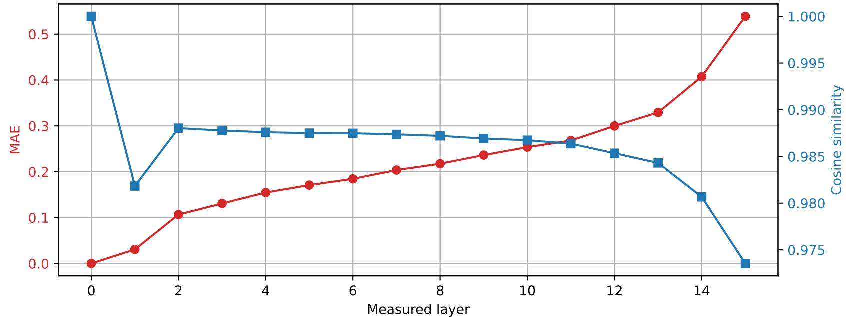
Llama-3.2-1B | Prompt 4 Spared layer 7 | Hybrid vs unquantized
