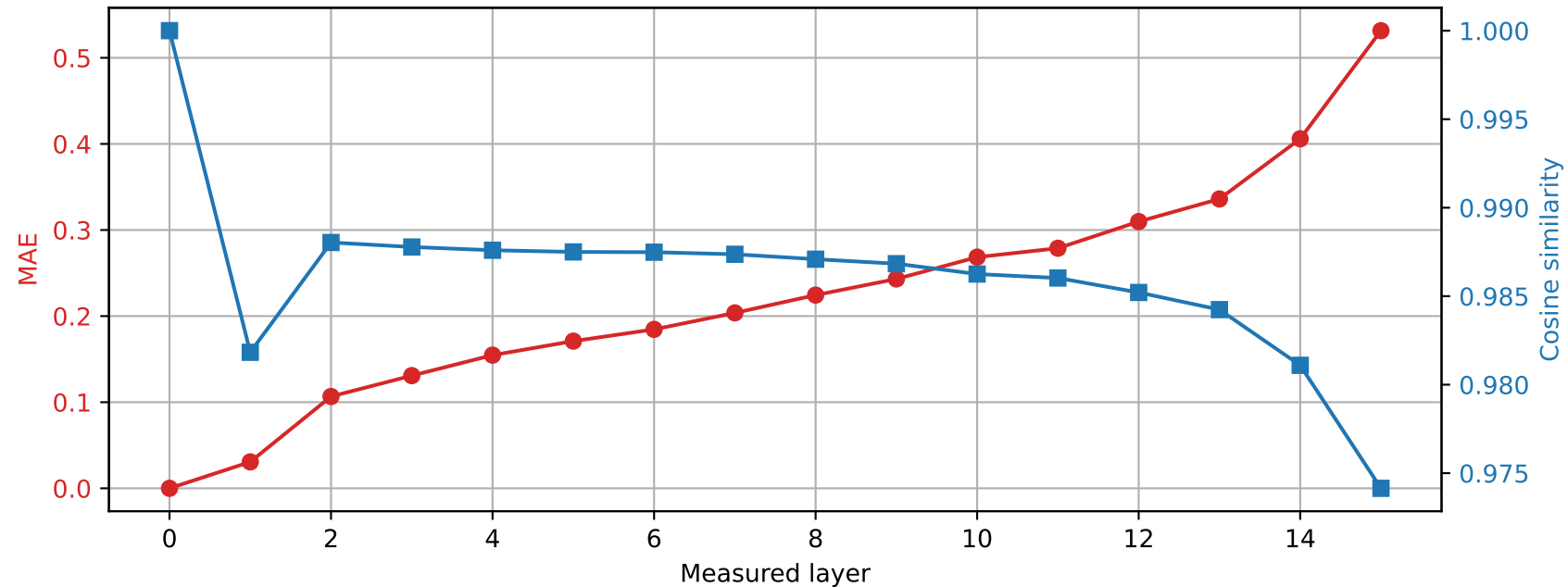
Llama-3.2-1B | Prompt 4 Spared layer 9 | Hybrid vs unquantized
