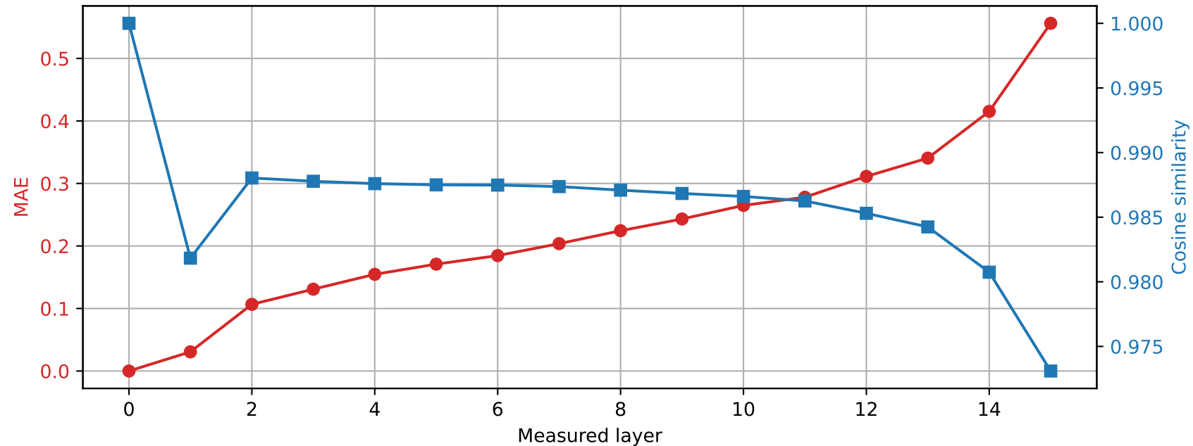
Llama-3.2-1B | Prompt 4 Spared layer 15 | Hybrid vs unquantized
