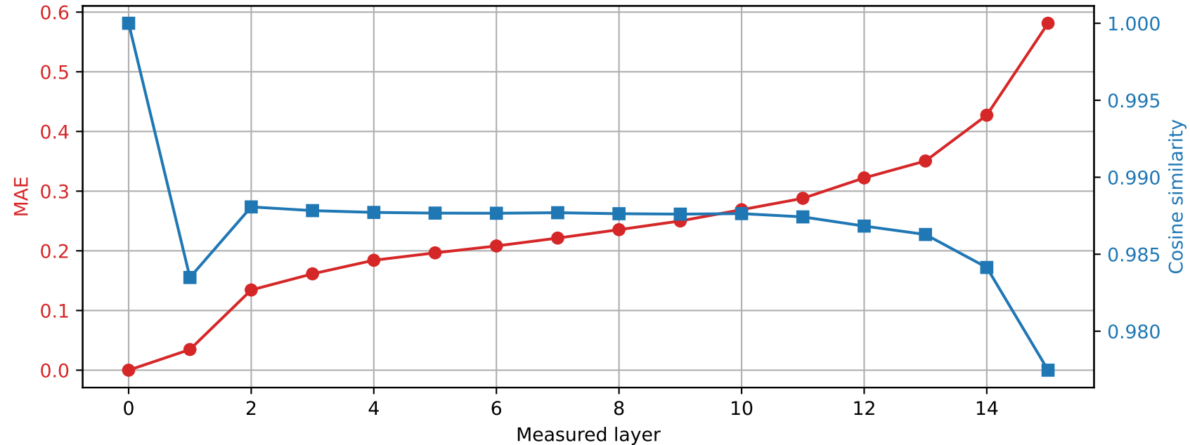
Llama-3.2-1B | Prompt 0 Spared layer 4 | Hybrid vs unquantized
