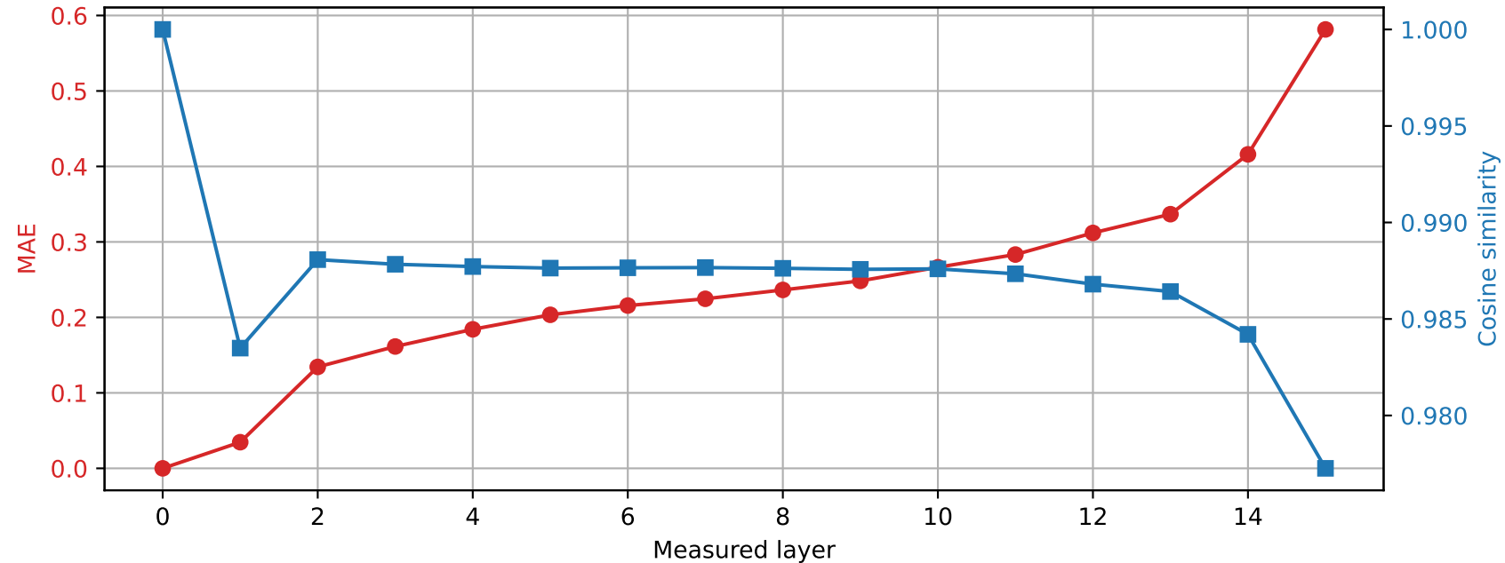
Llama-3.2-1B | Prompt 0 Spared layer 6 | Hybrid vs unquantized
