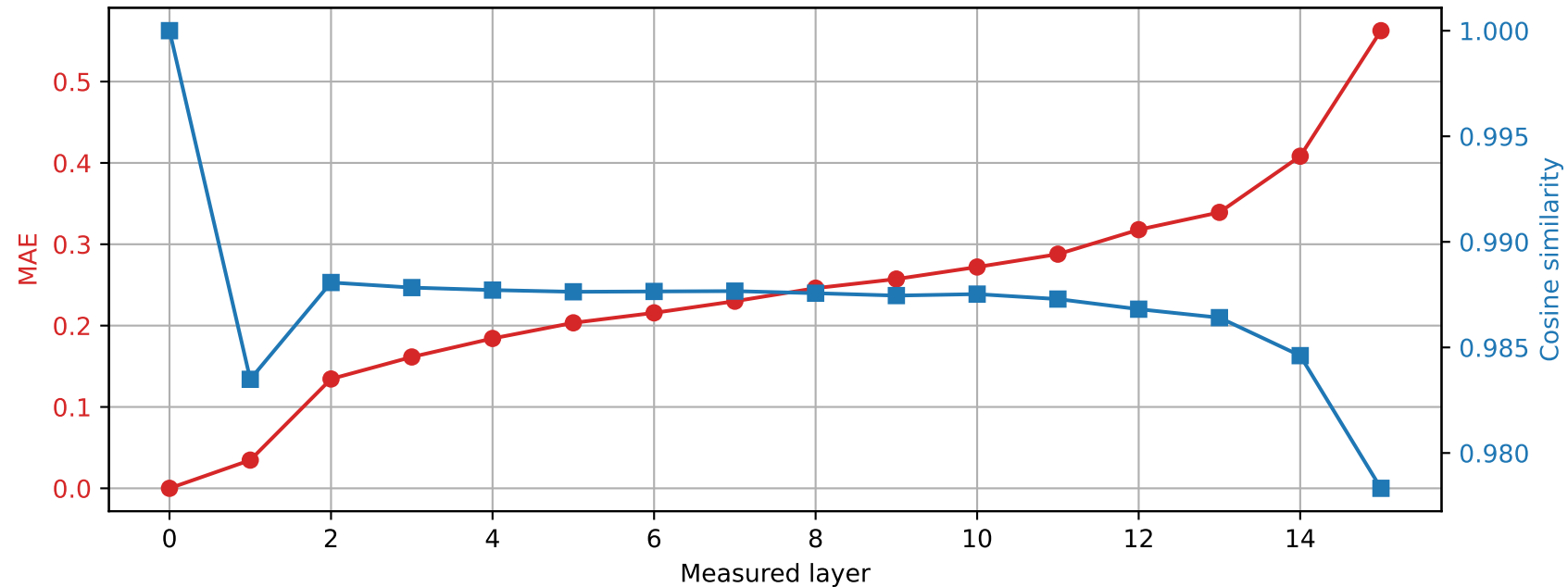
Llama-3.2-1B | Prompt 0 Spared layer 8 | Hybrid vs unquantized
