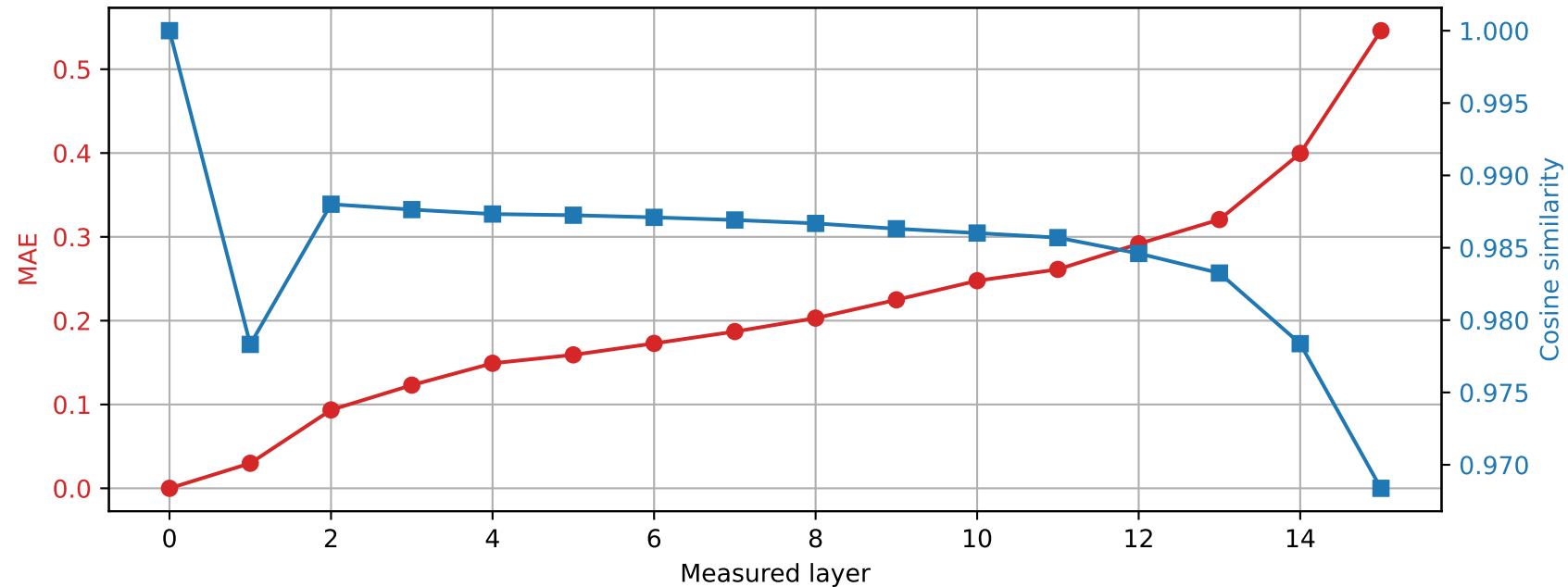
Llama-3.2-1B | Prompt 1 Spared layer 4 | Hybrid vs unquantized
